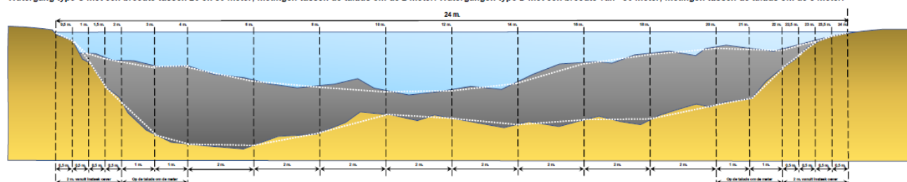
Figuur 2.7: Schematische weergave van de afstanden tussen de meetpunten in een dwarsprofiel.
