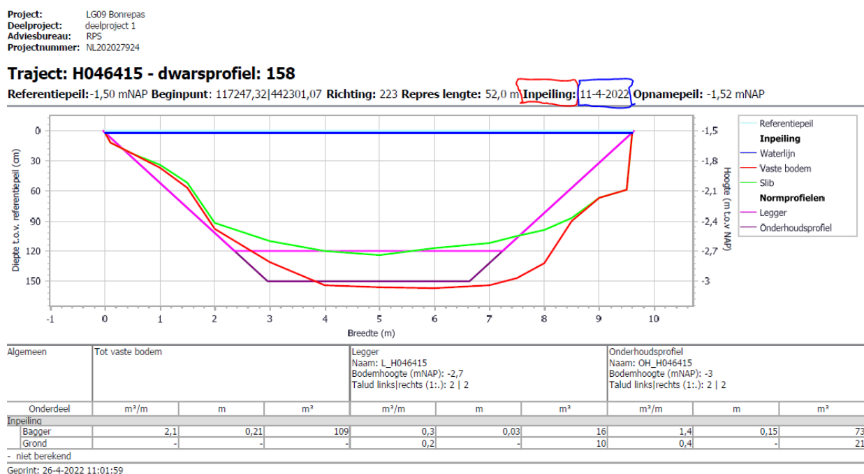
Figuur 2.13: Getekend profiel met dubbele Y-as.
