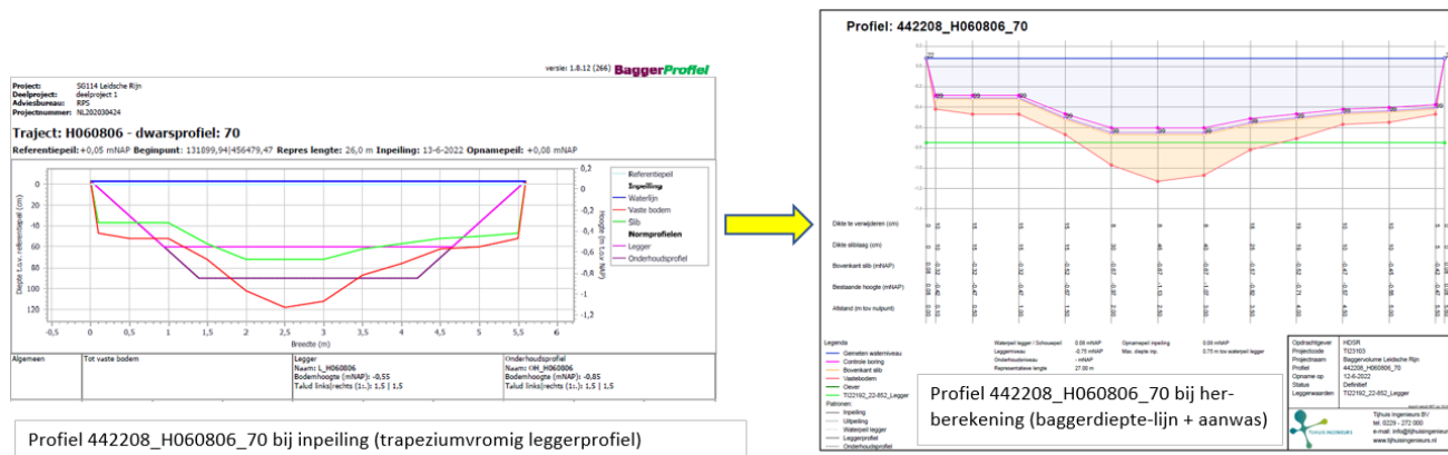
Figuur 3.5: links profiel 442208_H060806_70 met trapeziumvormig leggerprofiel bij inpeiling en rechts hetzelfde profiel met een horizontale (groene) te baggeren diepte-lijn en een paarse lijn voor de berekende slibaanwas.
