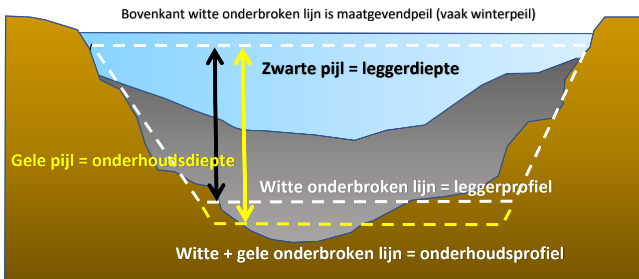
Figuur 2.9: Dwarsprofiel van een inpeiling met daarin getekend het legger- en onderhoudsprofiel.
