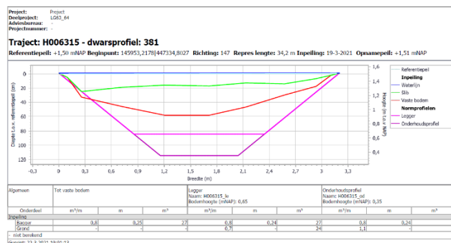
Figuur 2.10: Vaste bodem ligt boven de leggerdiepte.
