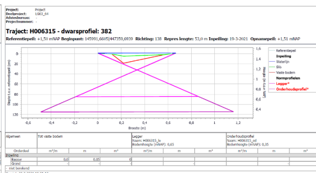
Figuur 2.11: Leggerprofiel past absoluut niet.
