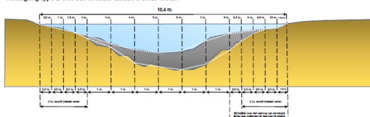
Watergang type B met een breedte tussen 5 en 20 meter.
