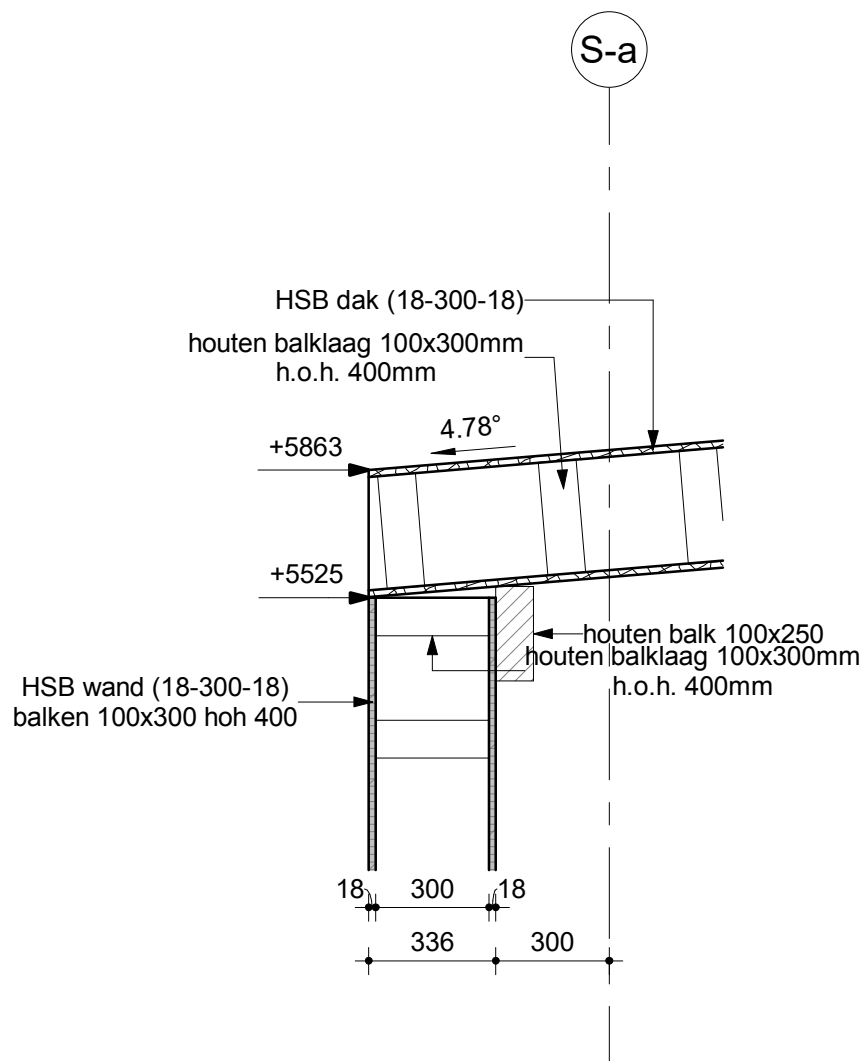
s.11 Detail Schaal: 1 : 20
