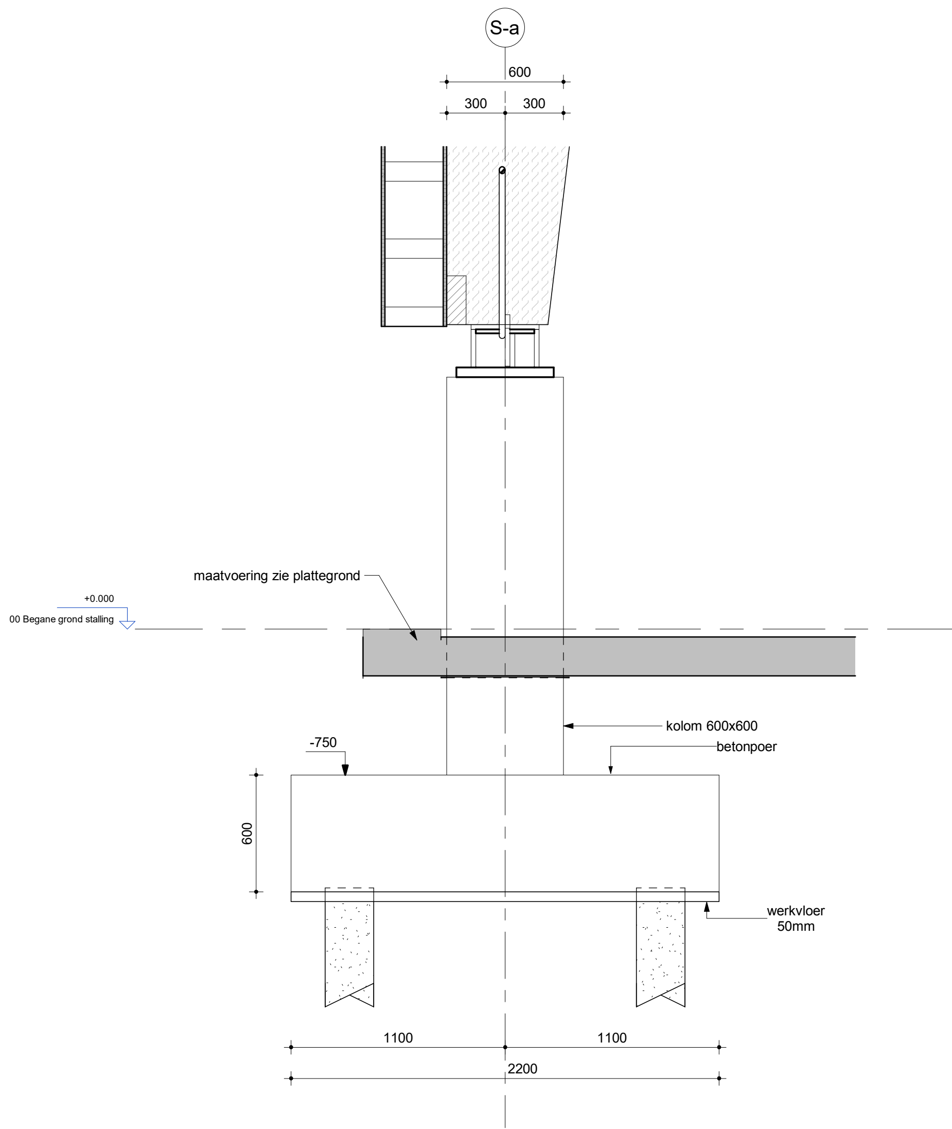
s.01 Detail Schaal: 1 : 20
