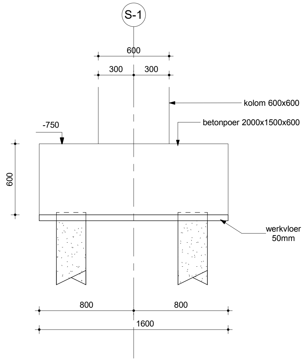
s.02 Detail Schaal: 1 : 20
