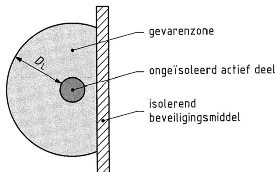
Figuur 2 — Begrenzing van de gevarenzone bij gebruikmaking van een isolerend beveiligingsmiddel, bijvoorbeeld met een beschermingsgraad IPXXB of IP2X
