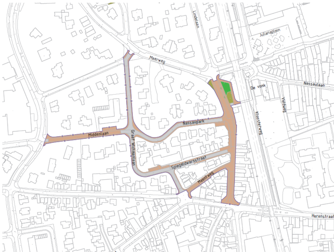
Figuur 1: Plangrenzen project Herinrichting Spiegelstraat
