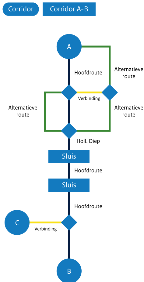
Figuur 12.1: Schematische weergave van een corridor
