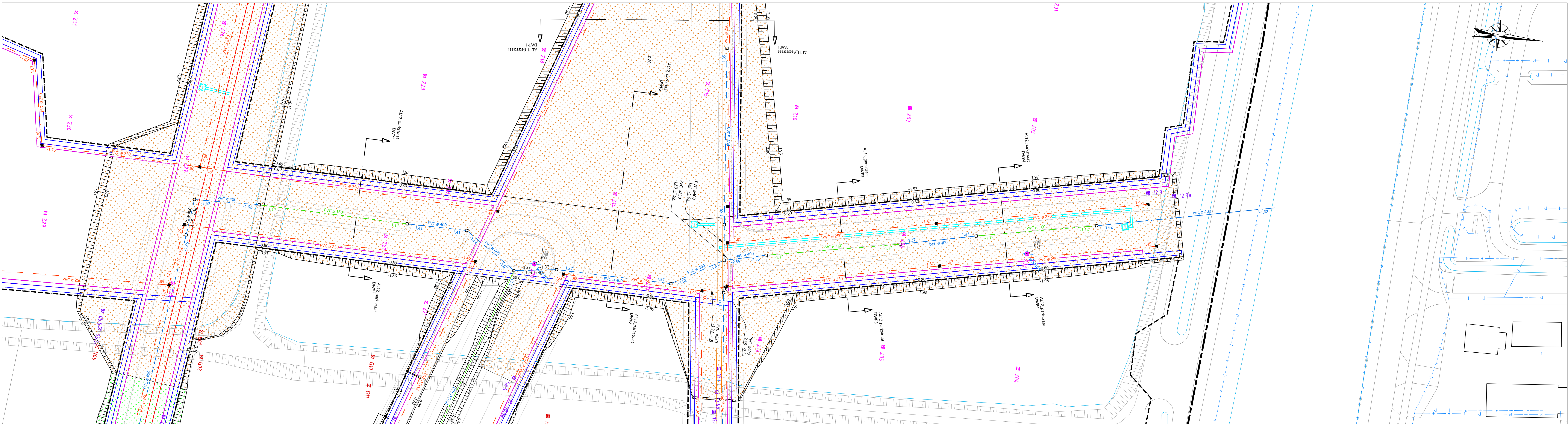
Situatie Parkstraat schaal 1:500
