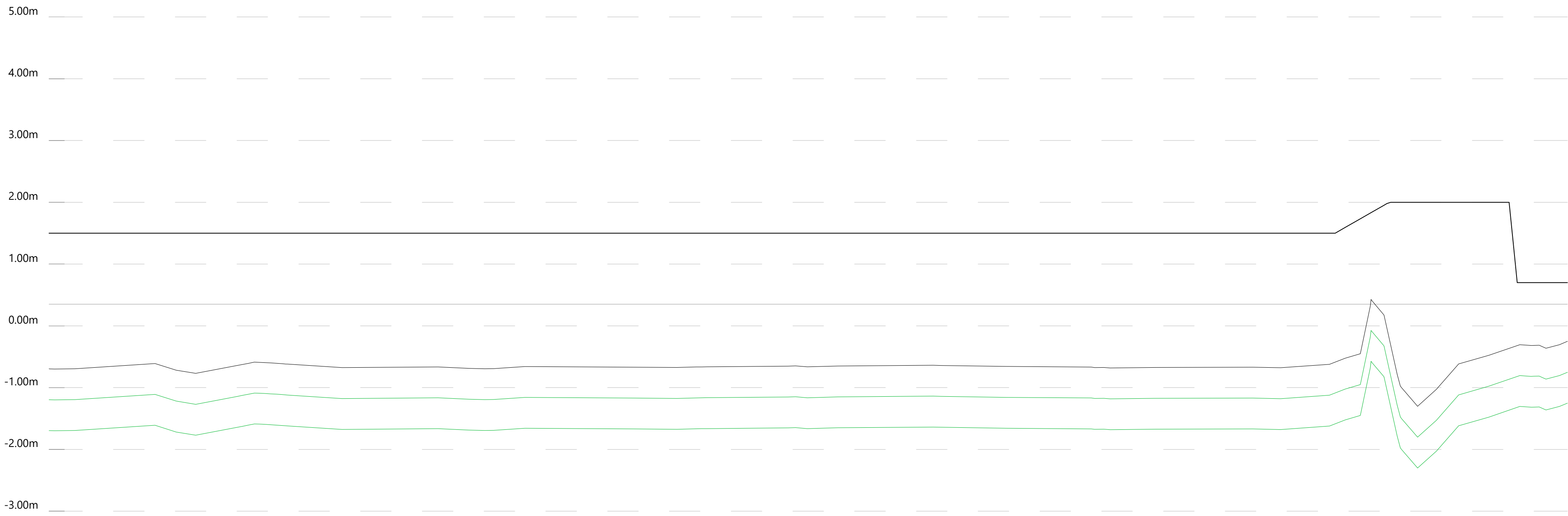
Lengteprofiel AL06_pionierspleinzuid Metreering 0 tot 246 Horizontale schaal 1:500 Verticale schaal 1:10
