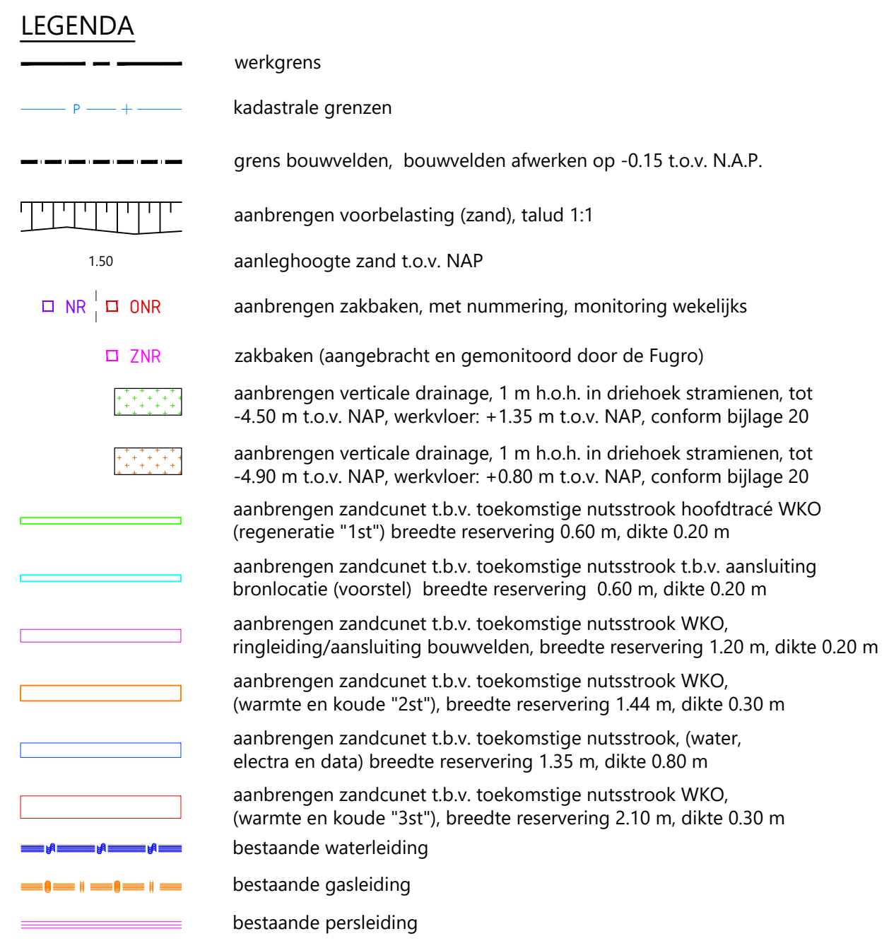
LEGENDA BRM/ONDERGRONDSE INFRA (buiten scope)
