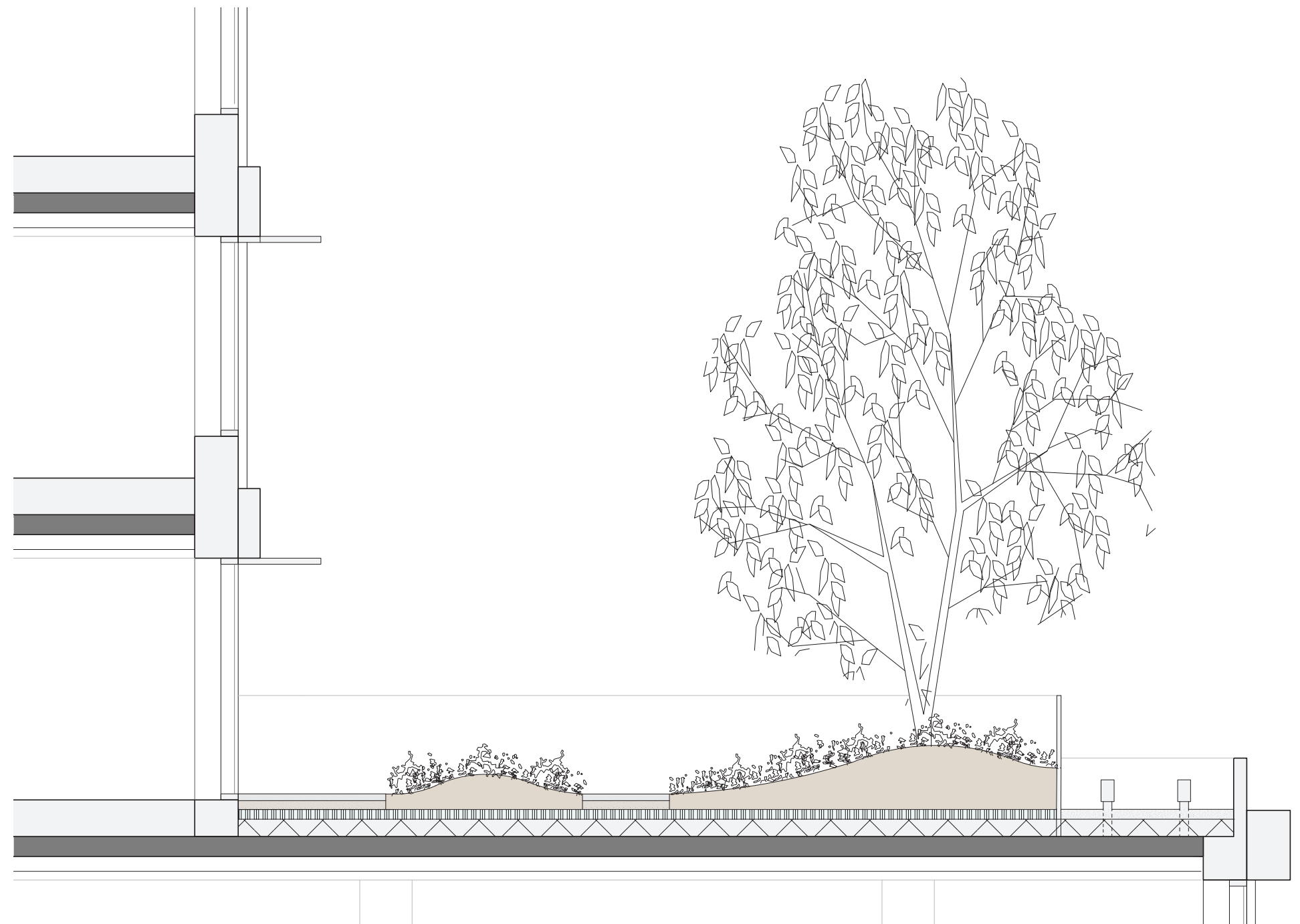
Doorsnede dakpakket daktuinen
