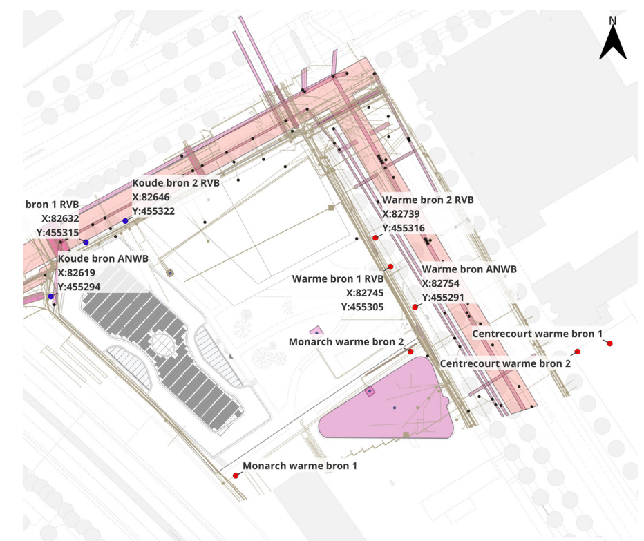
Posities bronnepunten WKO
