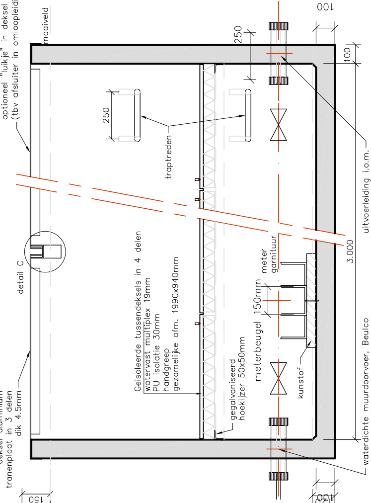
lengteboordsnede schaal 1:20
