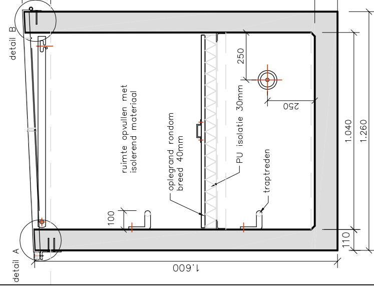
breedteboordsnede schaal 1:20
