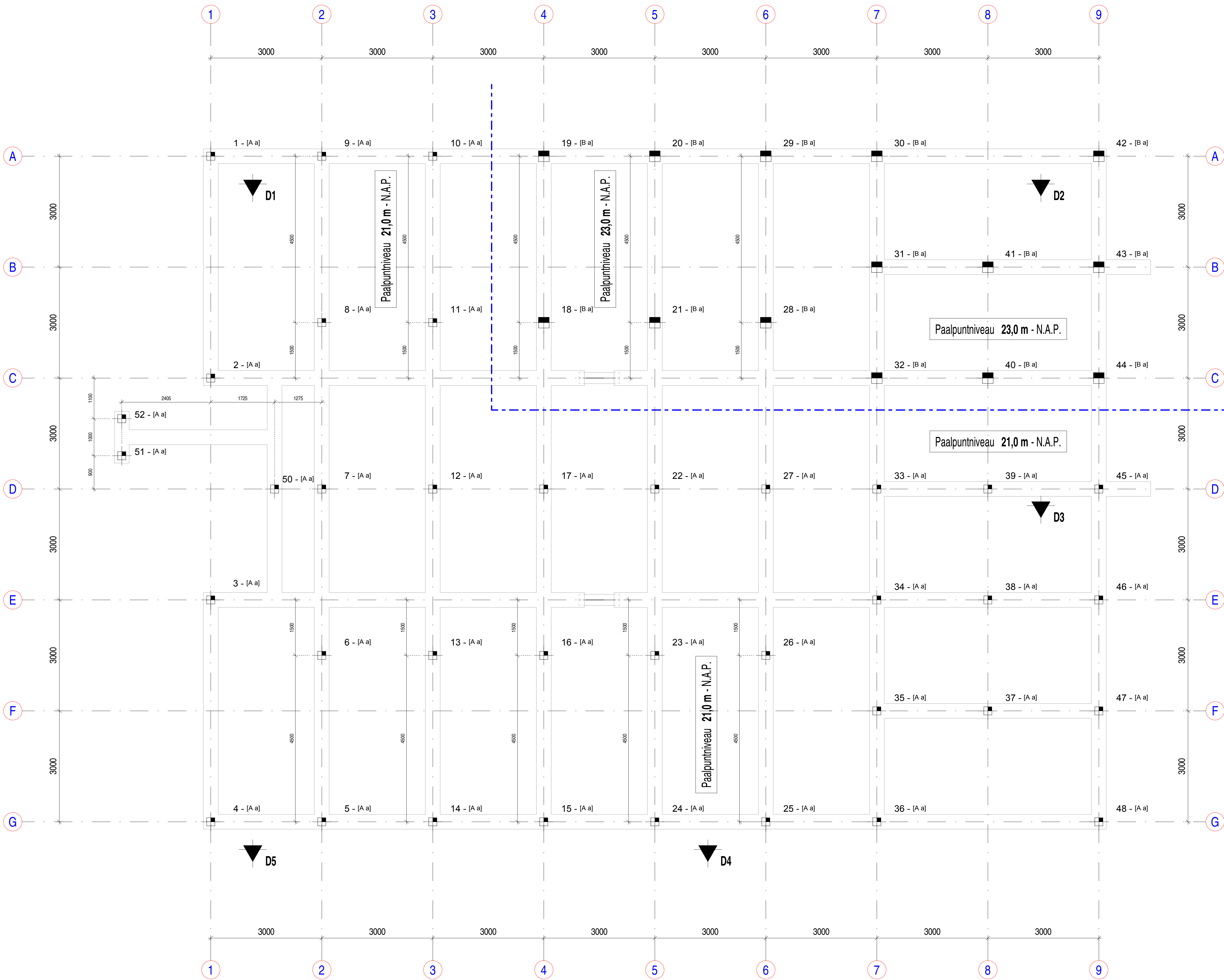
palenplan , Schaal: 1 : 50
