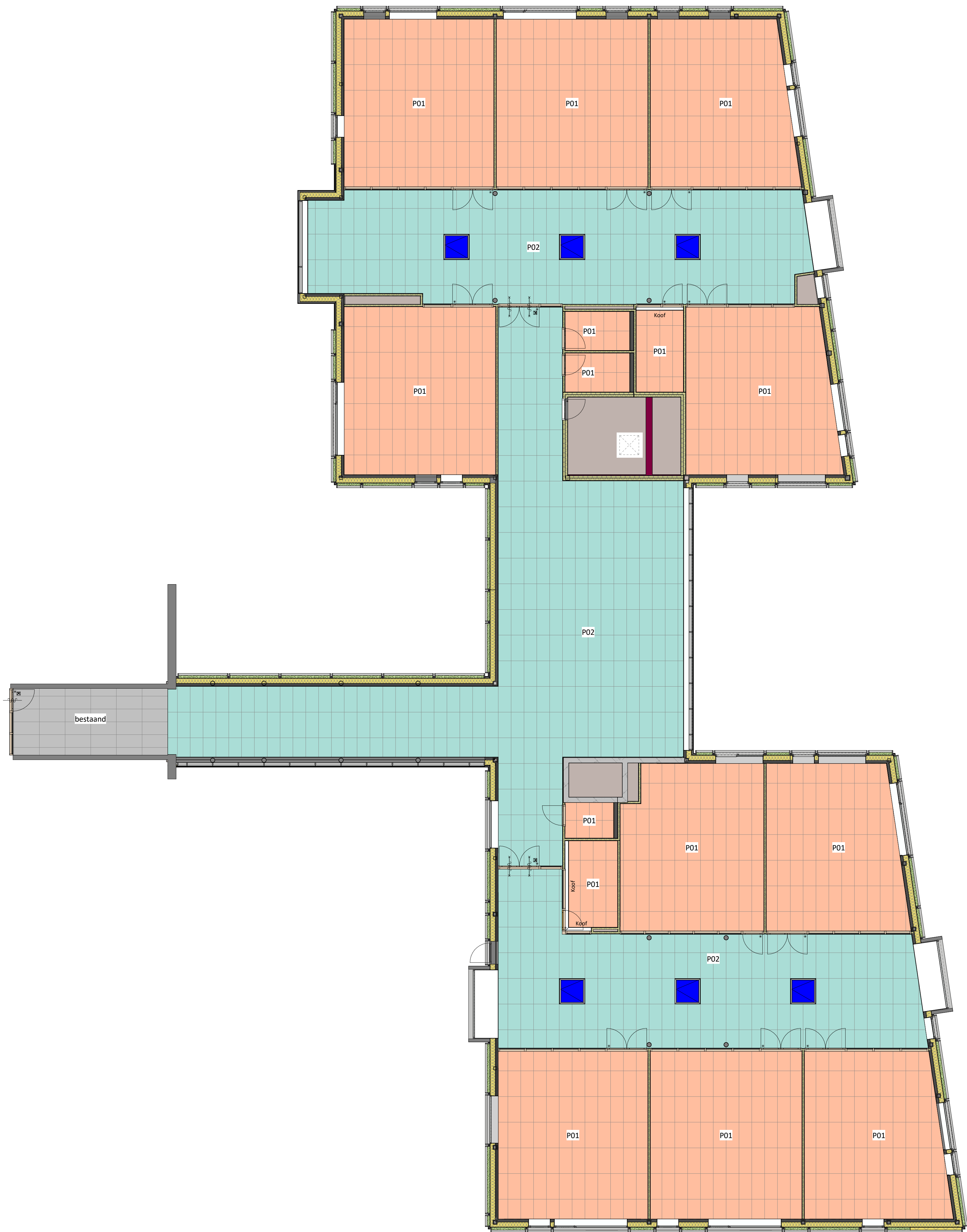
2 Eerste Verdieping 1 : 100
