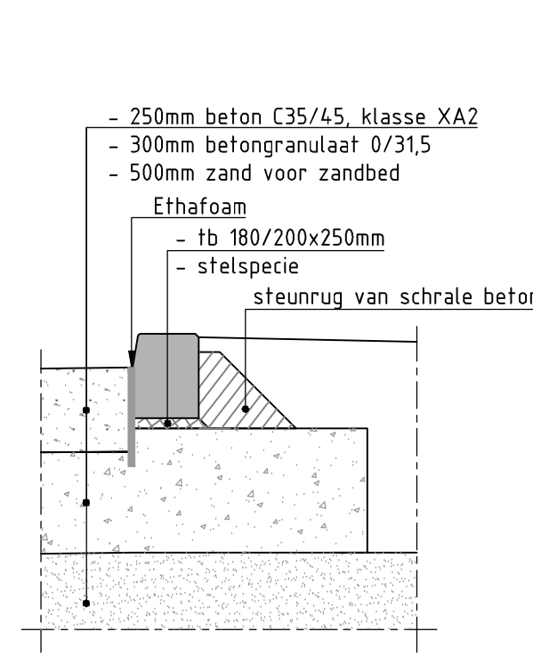
DETAIL: KANTOPSLUITING BETON SCHAAL 1 : 20
