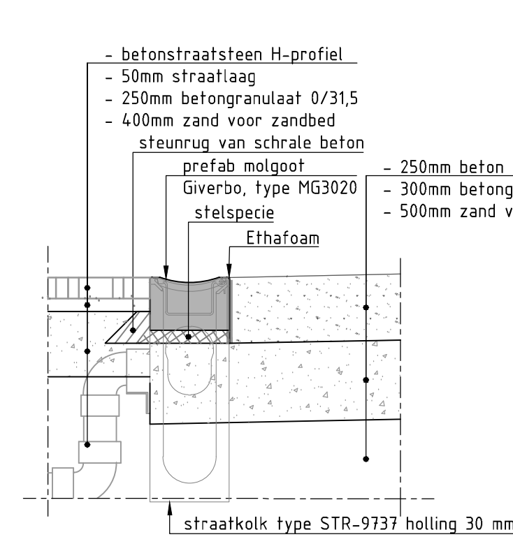
DETAIL: PREFAB GOOT BSS-BETON SCHAAL 1 : 20
