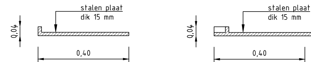
DETAIL: 1A - GELEIDERAIL SCHAAL 1 : 10
