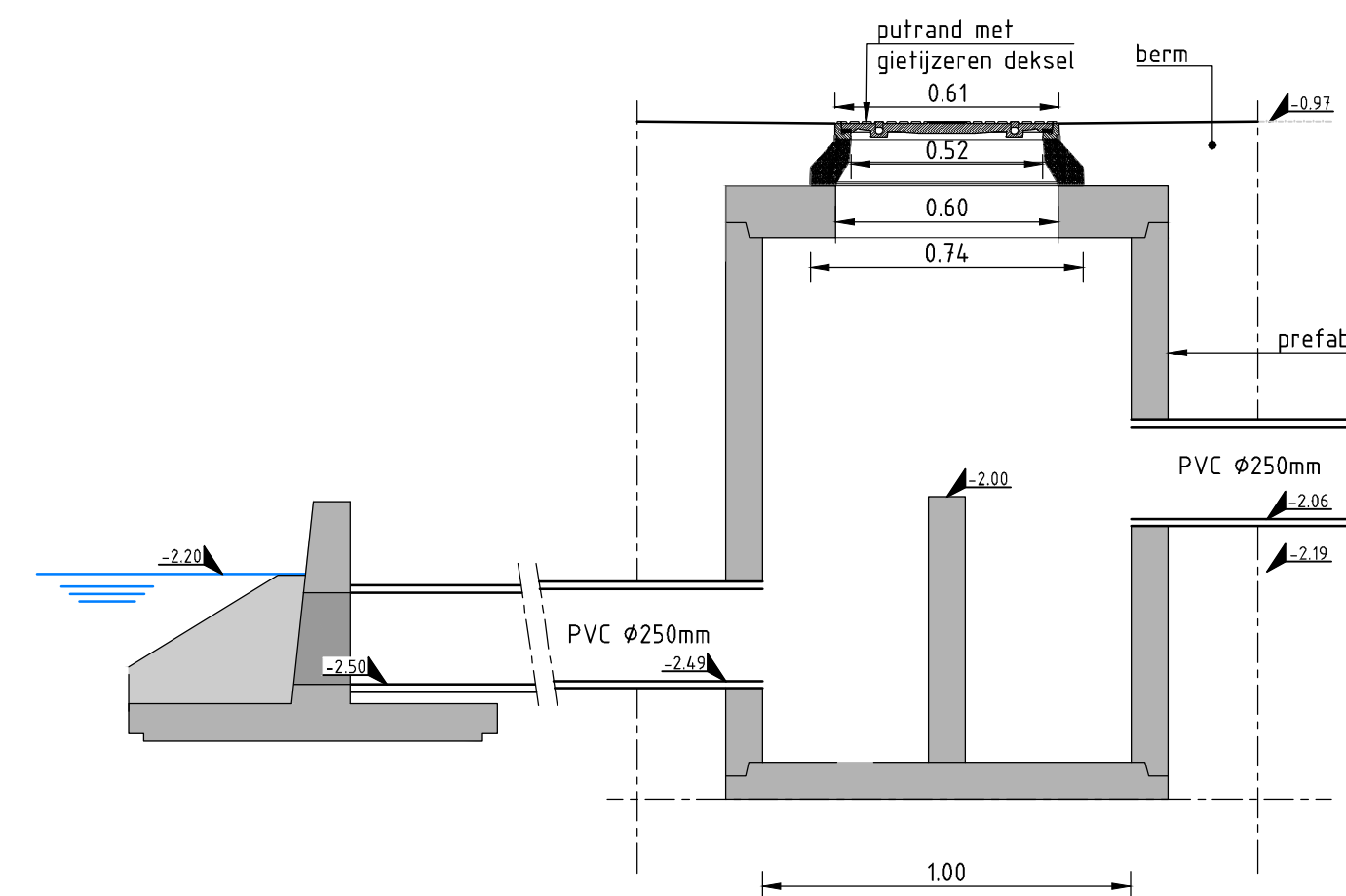
DETAIL: OVERSTORTPUT MET UITSTROOMBAC SCHAAL 1 : 20
