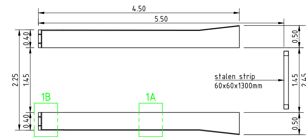
DETAIL: CONTAINER-GELEIDERAIL SCHAAL 1 : 50
