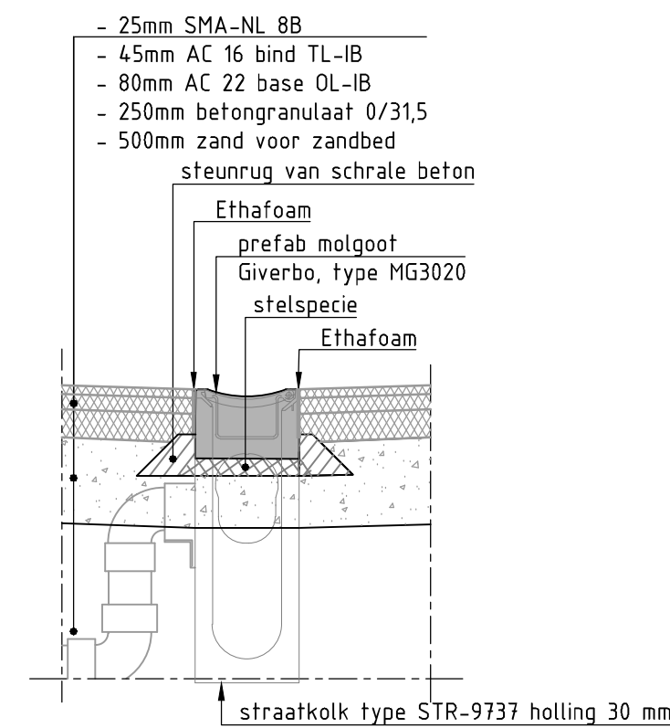
DETAIL: PREFAB GOOT ASFALT SCHAAL 1 : 20
