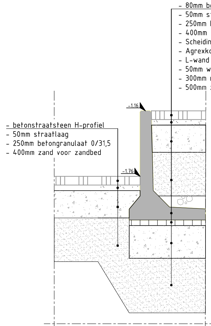
DETAIL: L-WAND BORDES SCHAAL 1 : 20
