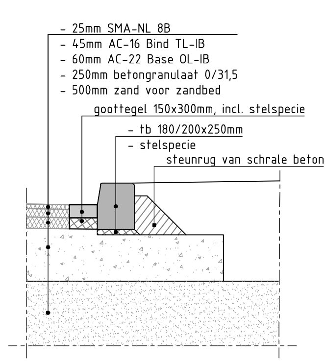
DETAIL: KANTOPSLUITING ASFALT SCHAAL 1 : 20
