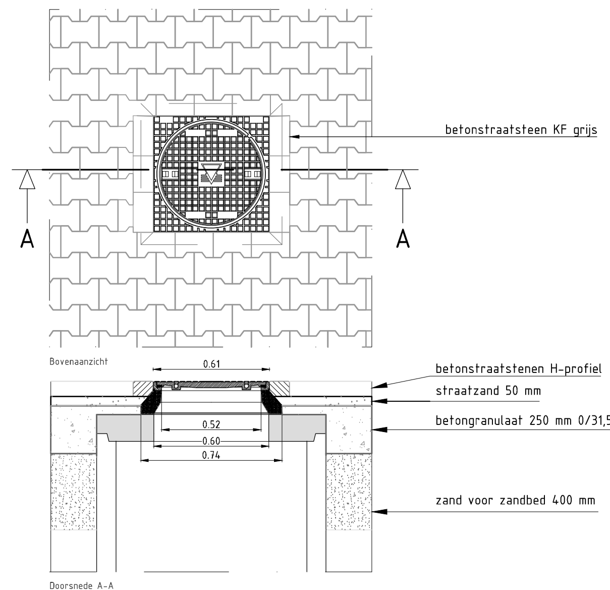
DETAIL: PUTDEKSEL IN ELEMENTENVERHARDING SCHAAL 1 : 20
