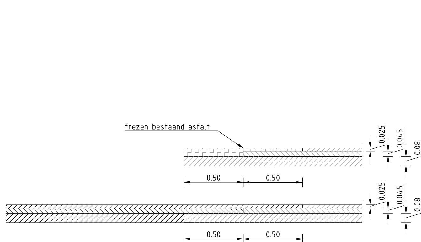
DETAIL: FREESTRAP SCHAAL 1:20
