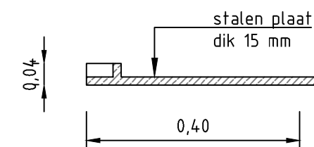
DETAIL: 1B - GELEIDERAIL SCHAAL 1 : 10
