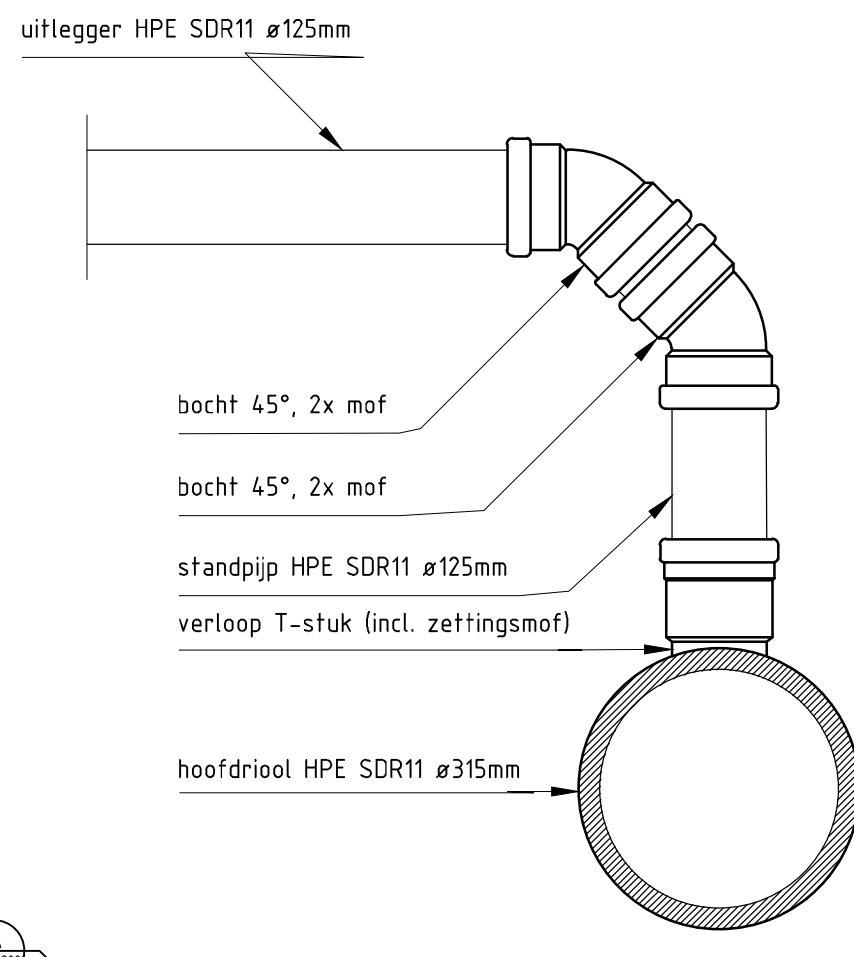
DETAIL: AANSLUITING OP HPE HOOFDRIJOL SCHAAL 1 : 10
