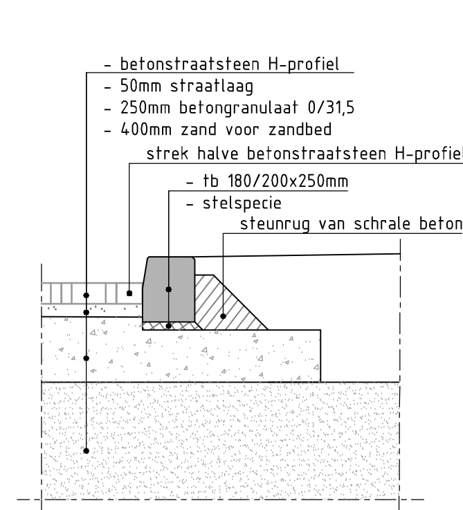
DETAIL: KANTOPSLUITING BSS SCHAAL 1 : 20
