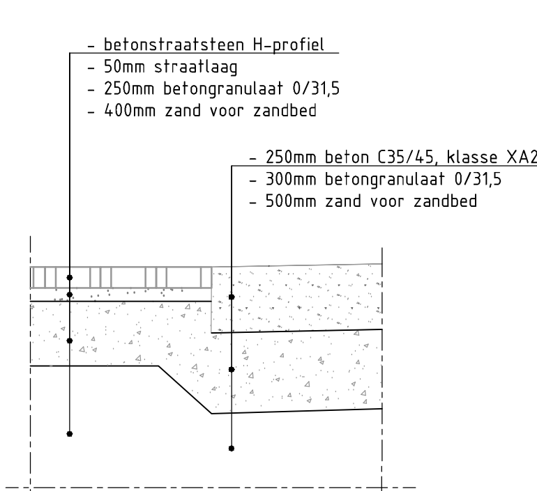
DETAIL: AANSLUITING BETON-BSS SCHAAL 1 : 20
