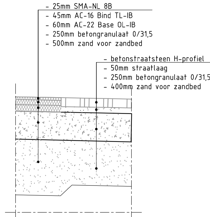
DETAIL: AANSLUITING ASFALT-BSS SCHAAL 1 : 20
