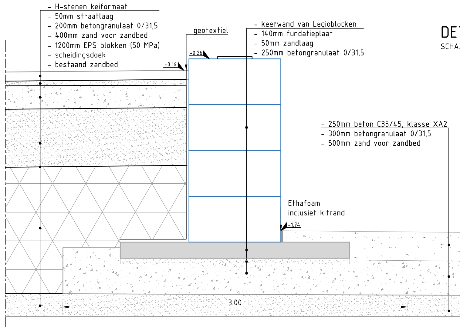
DETAIL: KEERWAND UIT LEGIOBLOCKEN SCHAAL 1 : 20
