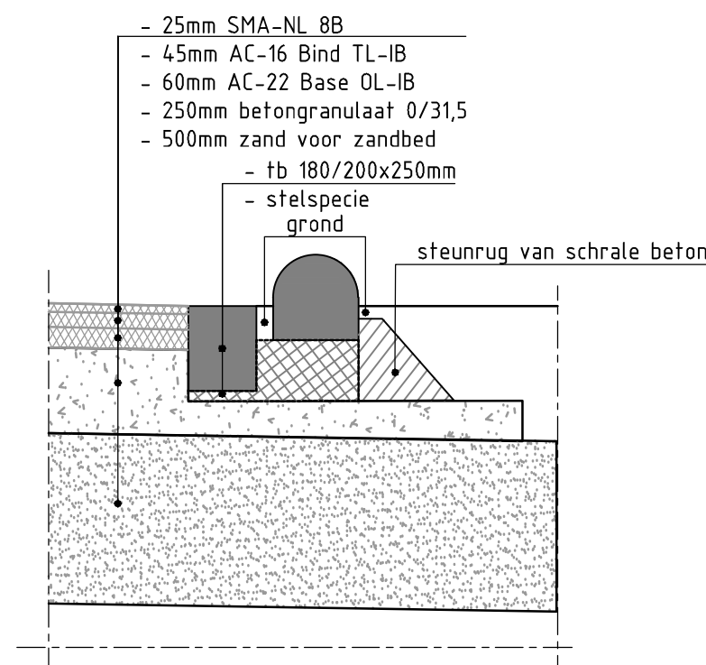
DETAIL: KANTOPSLUITING MET STOOTBAND SCHAAL 1 : 20
