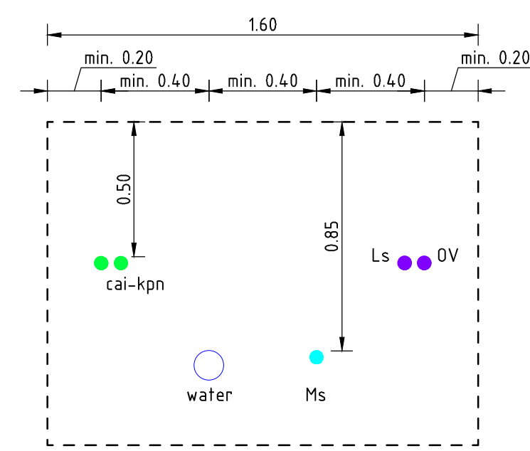
DETAIL: PRINCIPEPROFIEL K&L TRACÉ SCHAAL 1 : 20
