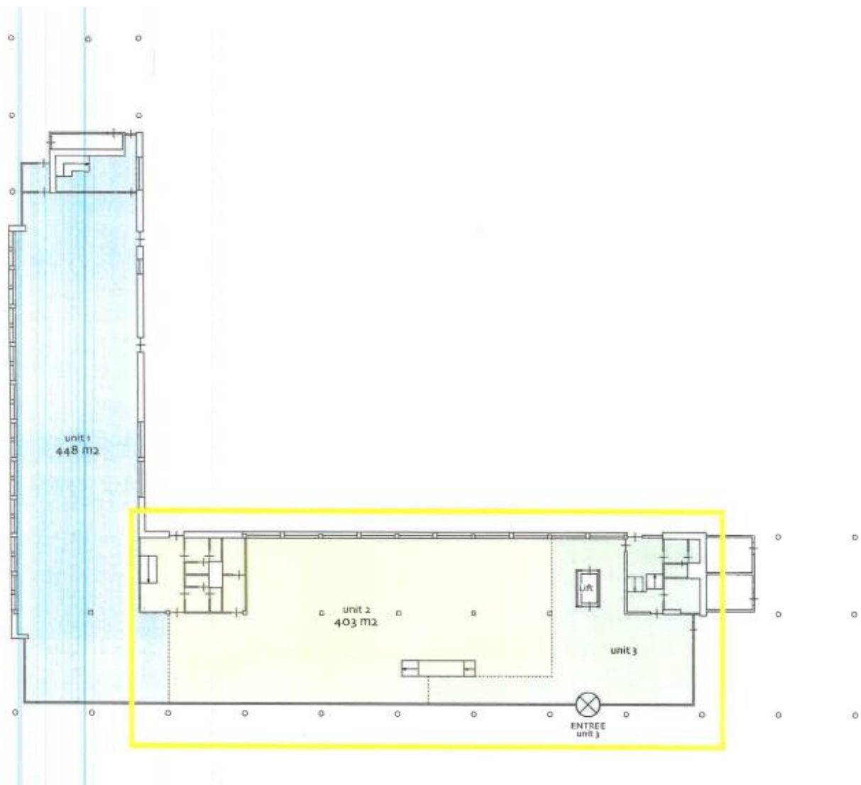
Begane grond
