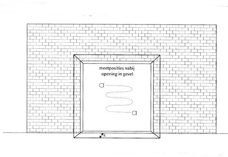
FIGUUR B.4.2 Bronsterktemeting van een open deur van een bedrijf; de bron wordt als een vlakke bron beschouwd
