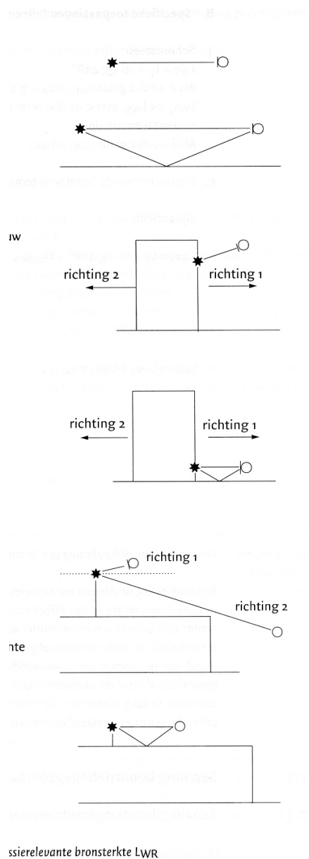
FIGUUR A.7.5 Voorbeelden van de berekening van de immissierelevante bronsterkte L_{WR}
