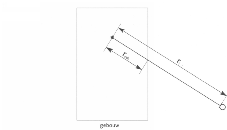
FIGUUR C.4.8 Bodemverzwakking boven dakvlakken (bovenaanzicht)
