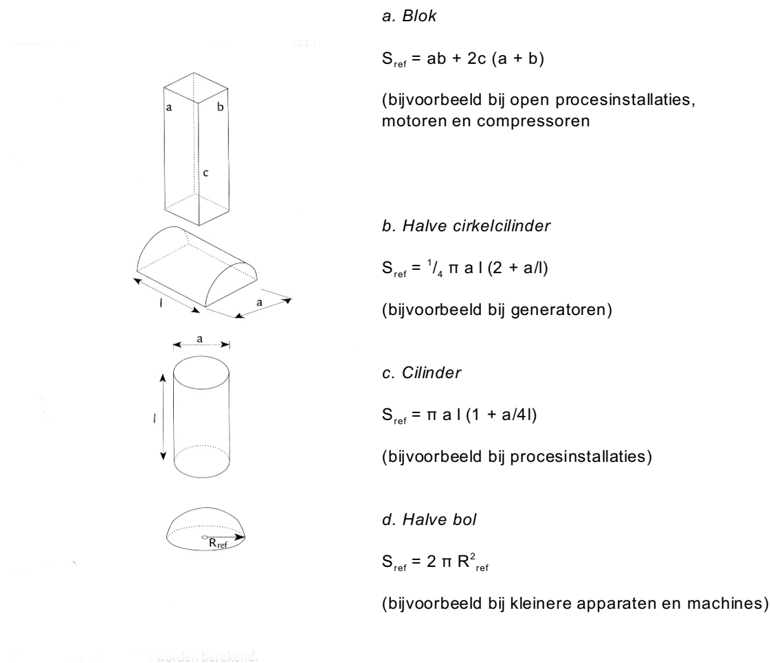
FIGUUR B.4.1 Vormen van referentieliĳaamen
