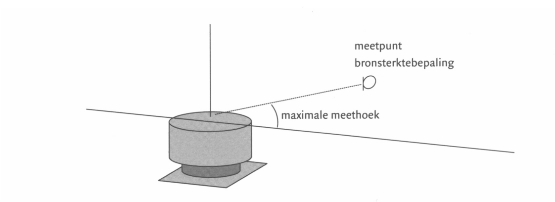
FIGUUR D.5 Meetposities rond ventilator
