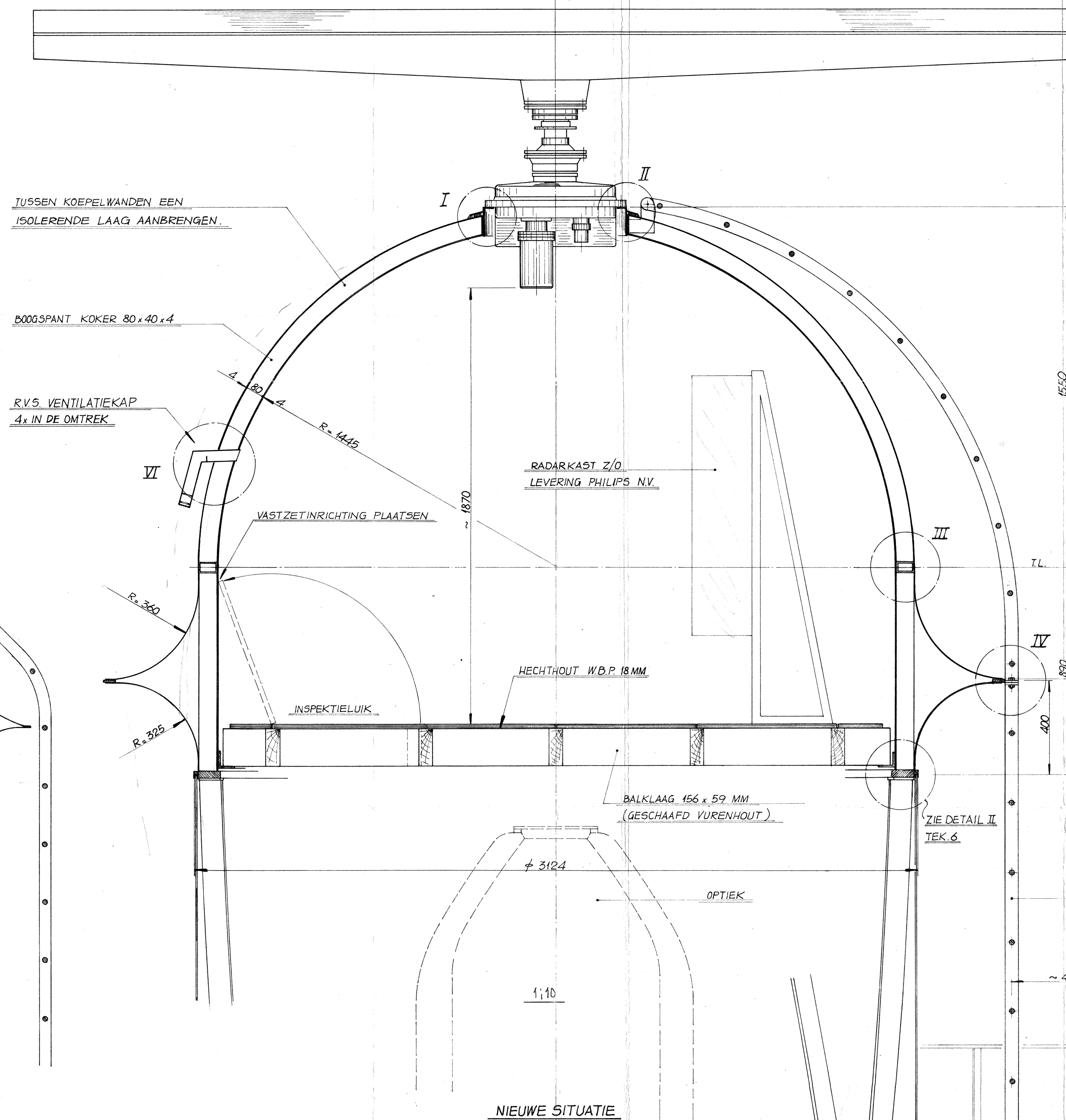
NIEUWE SITUATIE
