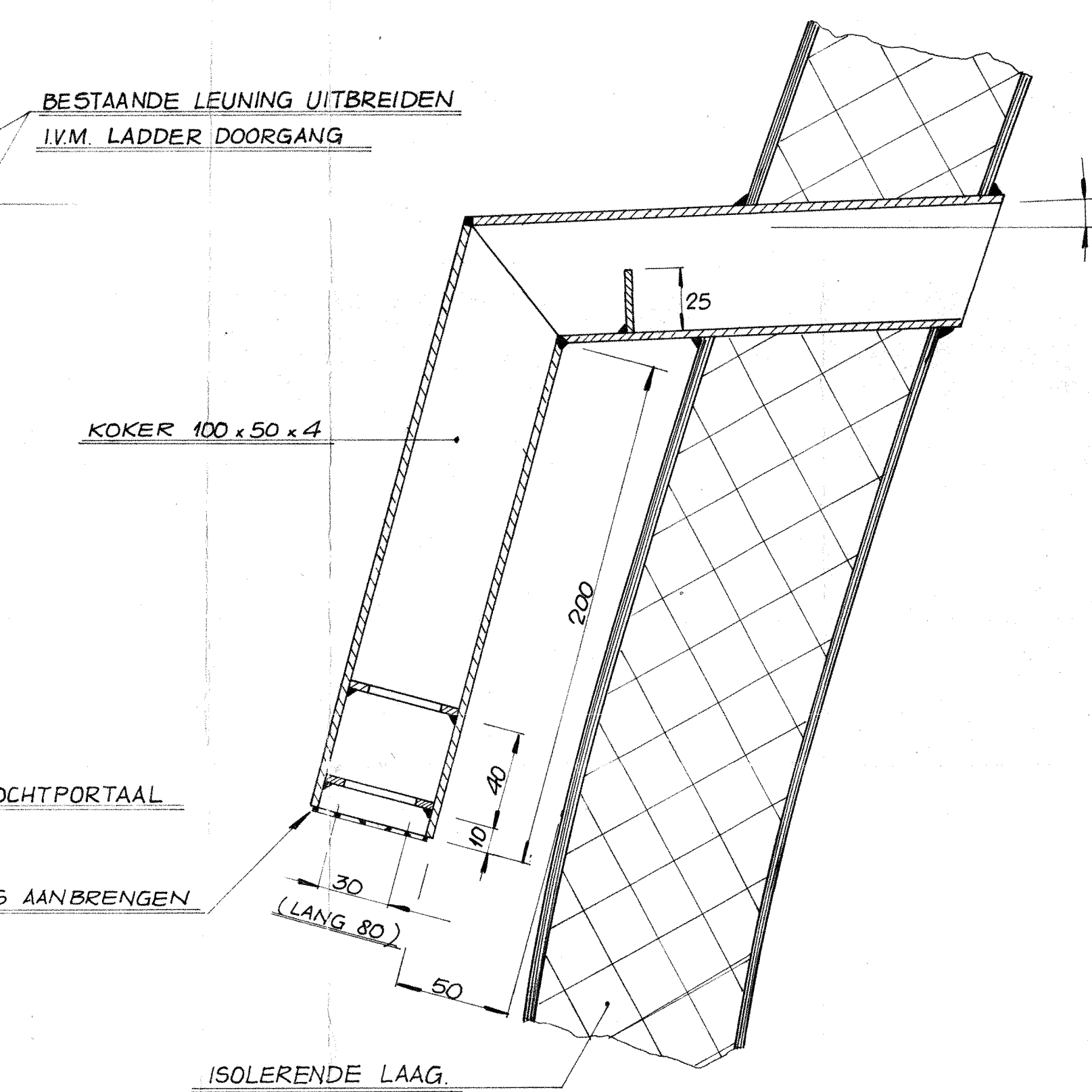
DETAIL VI
