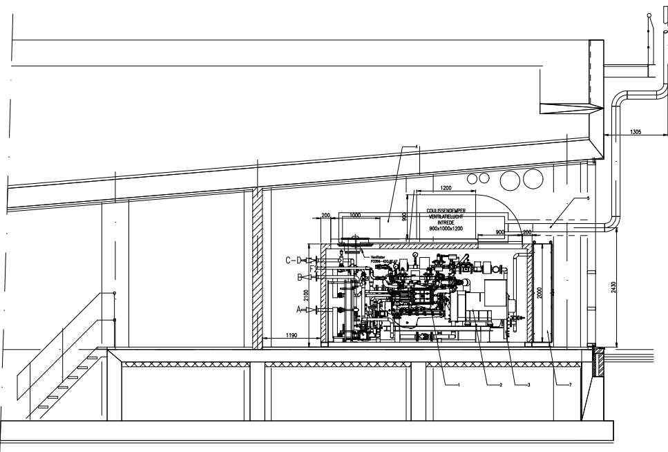
DOORSNEDE A-A
