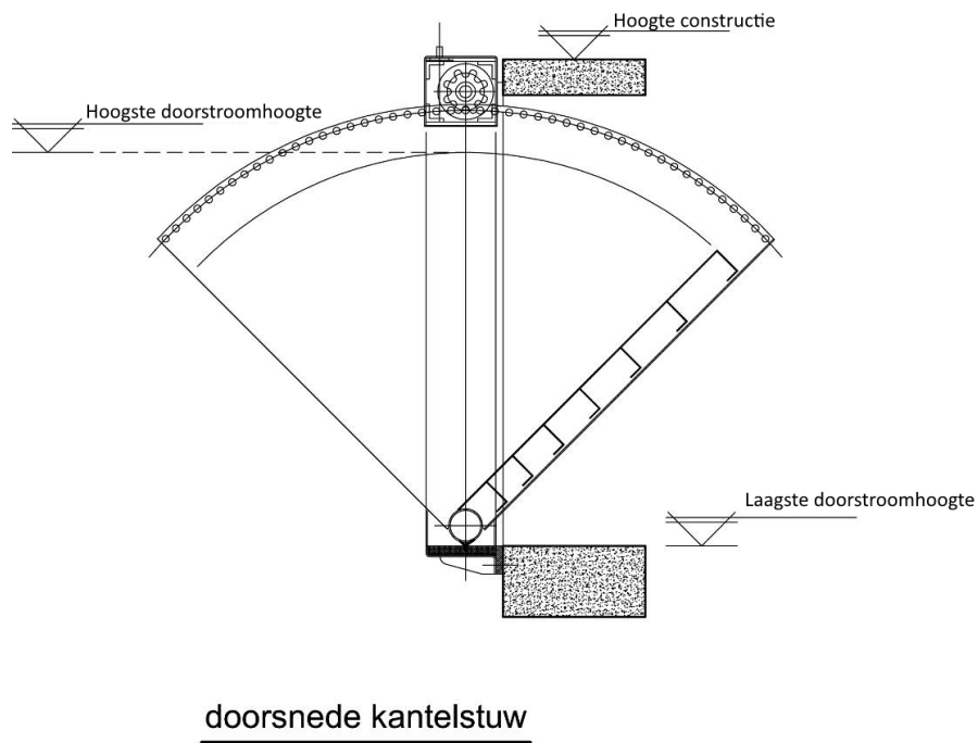
Figuur 8-29: Kantelstuw
