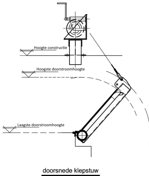
Figuur 8-30: Klepstuw
