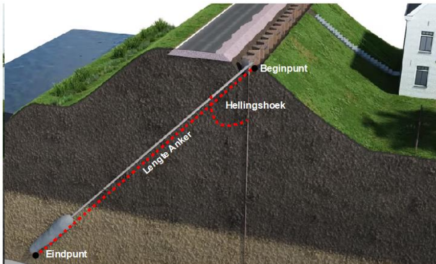
Figuur 8-12: Zijaanzicht anker
