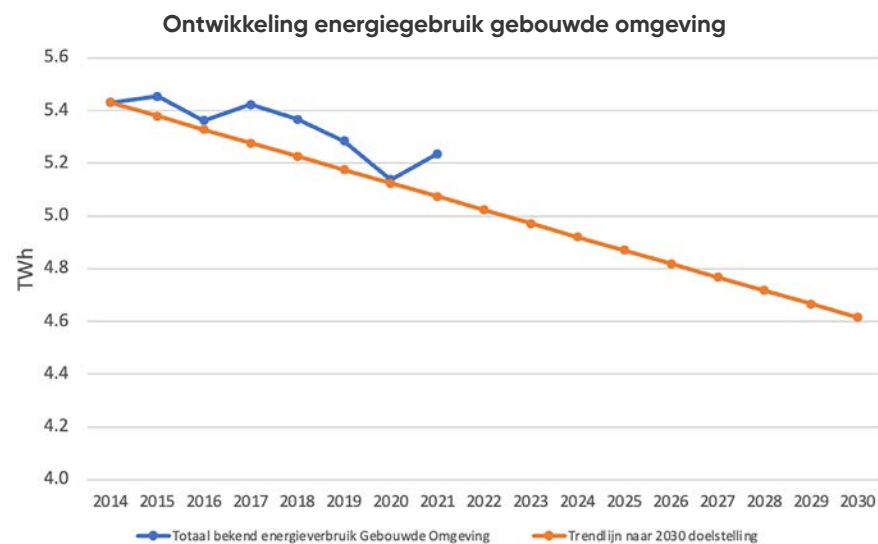
Figuur 3: Ontwikkeling energieverbruik gebouwde omgeving RES Holland Rijnland van 2014 tot 2020. In 2020 lag Holland Rijnland op koers, maar in 2021 vanwege de relatief koude winter is de vraag naar aardgas zowel in woningen, commerciële als publieke diensten gestegen.
