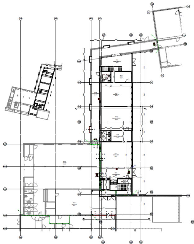
PLATTEGROND - BEGANEGROND
