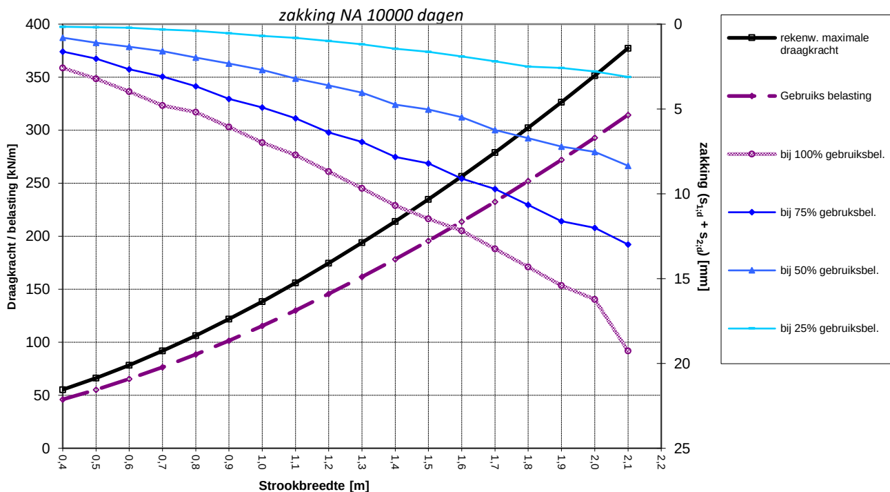
Figuur 3 Draagkracht-last-zakkingsgrafiek
