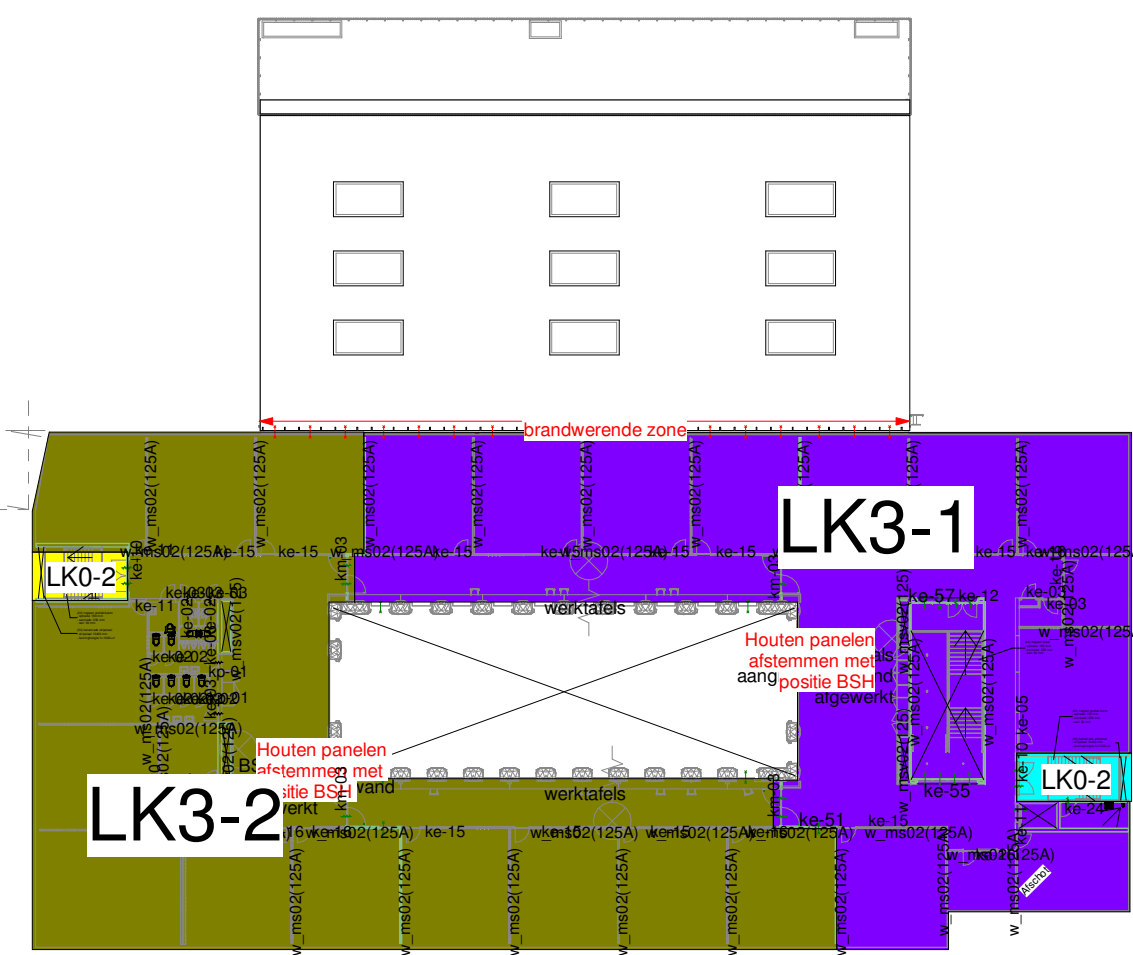
Principe verdelkast verdeling
