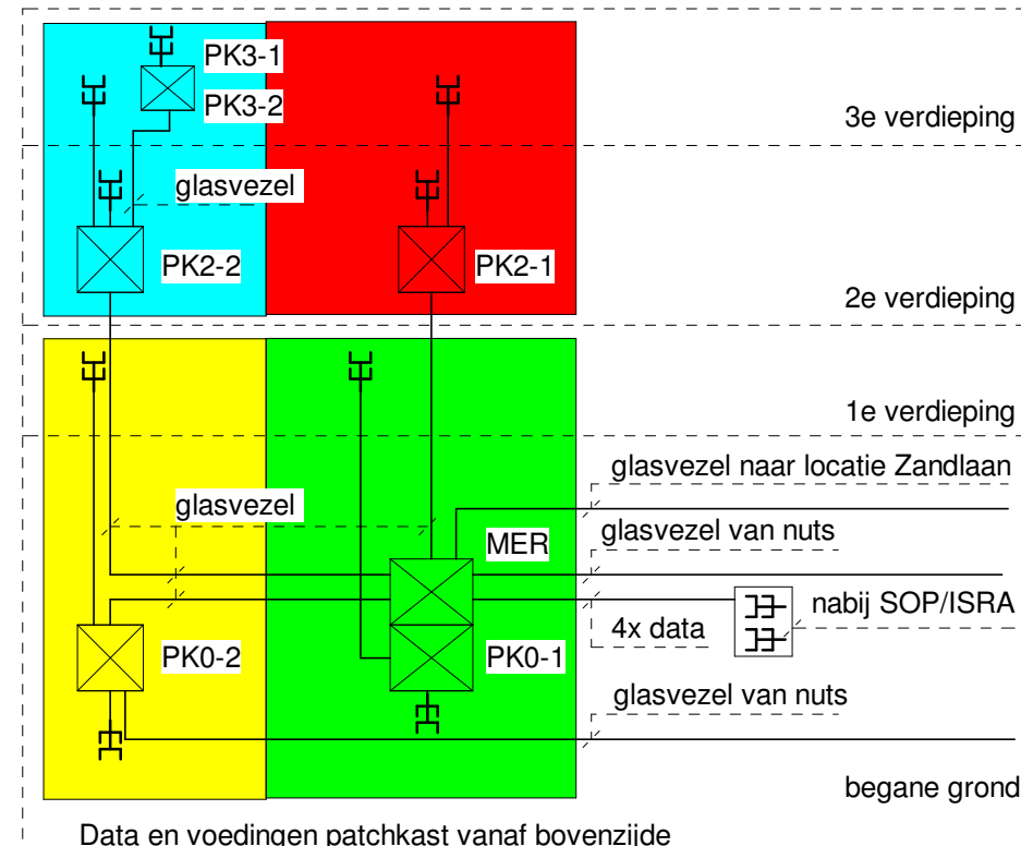
Principe blokschema data installatie
