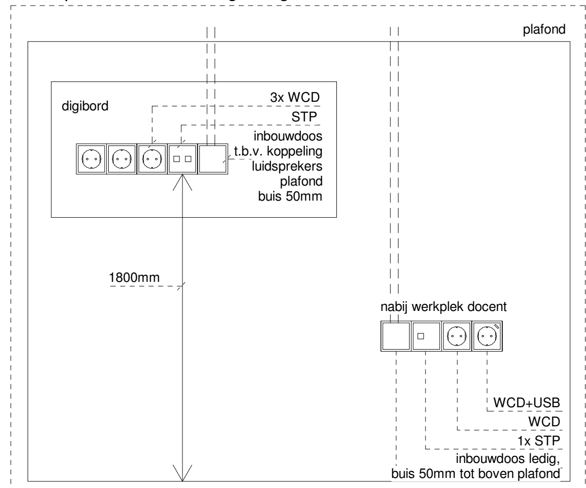
Principe detail voorzieningen digibord:
