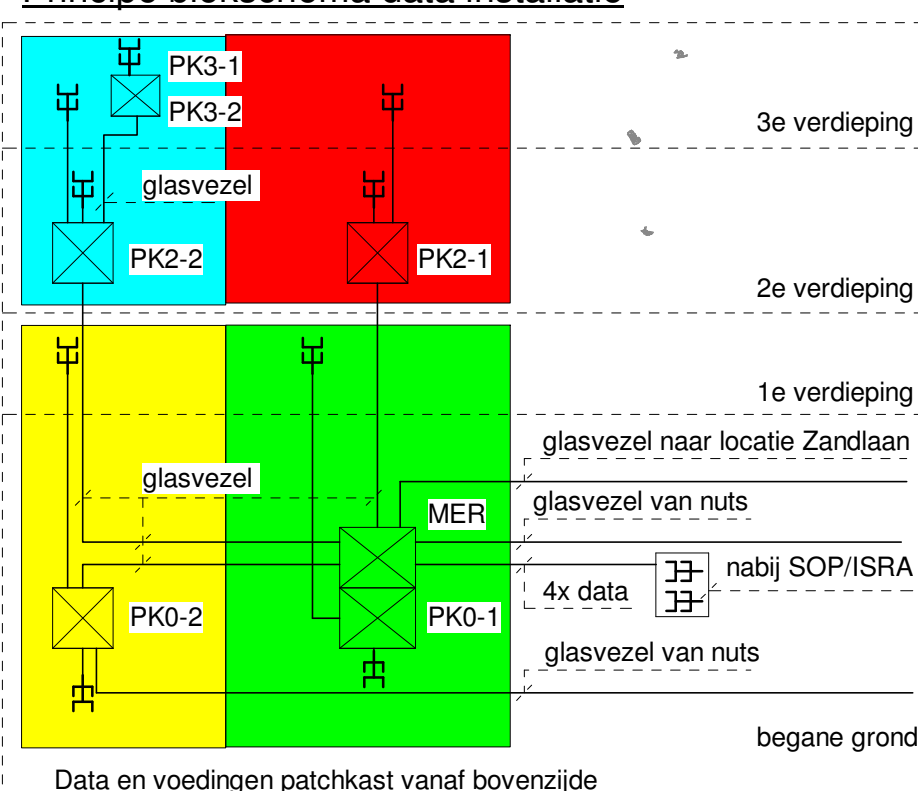
Principe blokschema data installatie
