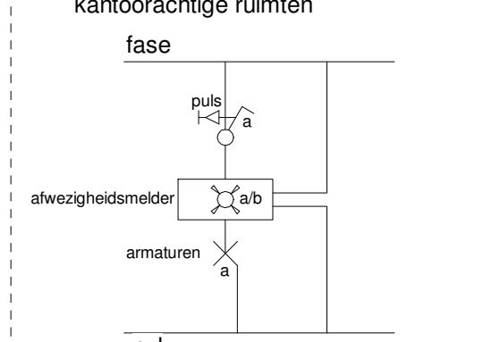
Principe detail lichtschakeling kantoorachtige ruimten
