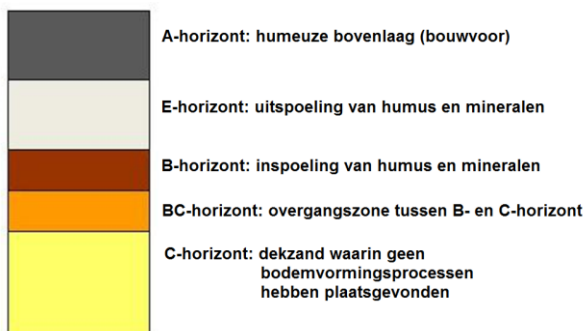
Afbeelding 14. Schematische voorstelling van een podzolbodem
