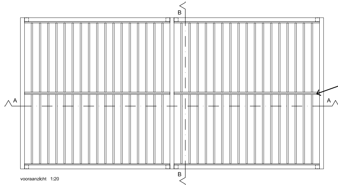
vooraanzicht 1:20
