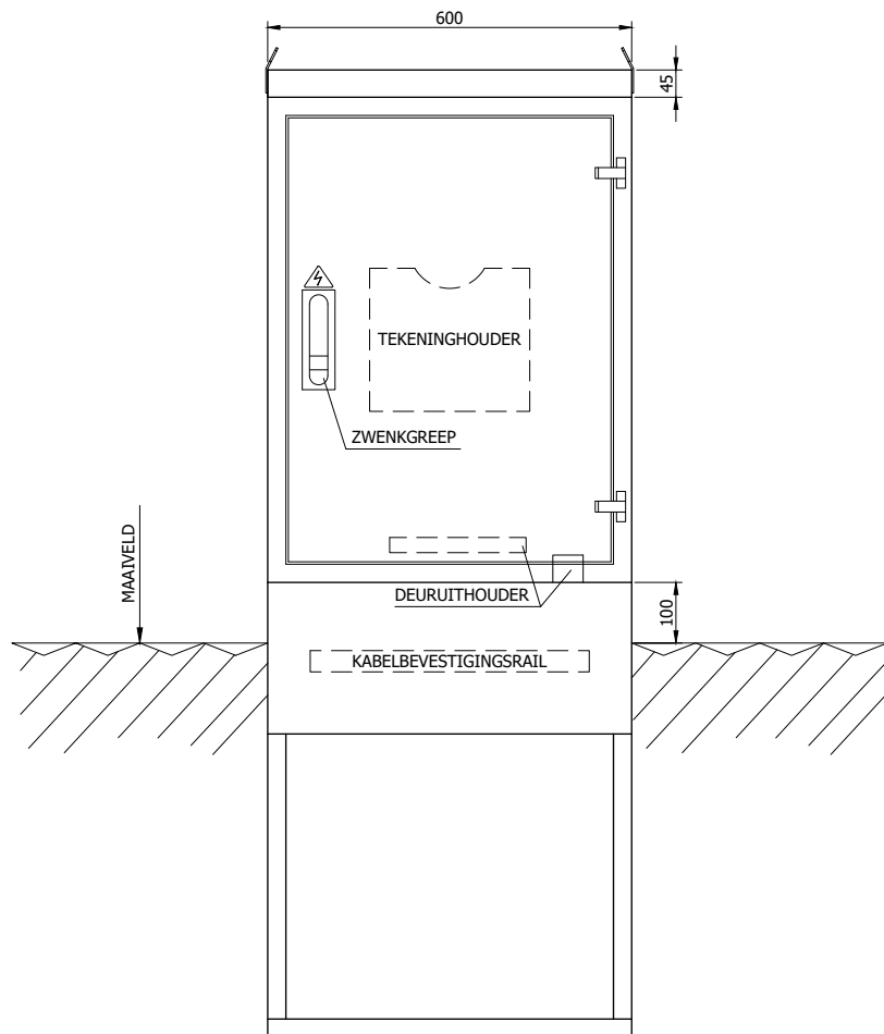
VOORAANZICHT
