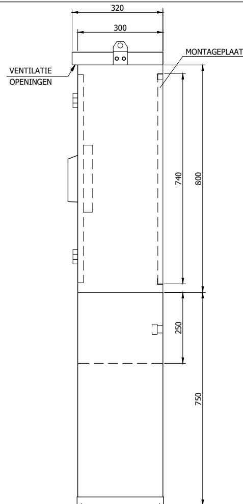
ZIJAAANZICHT RECHTS
