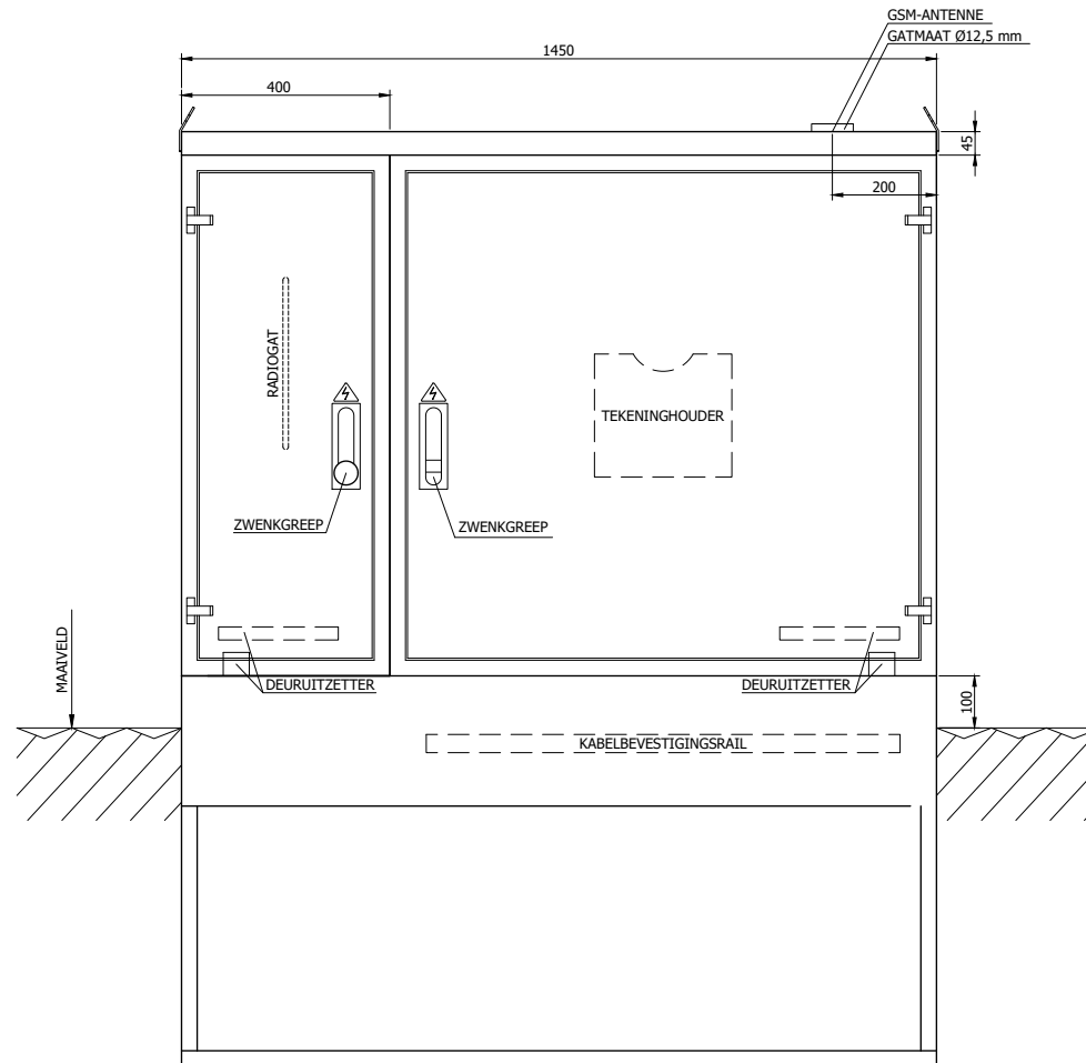
VOORAANZICHT
