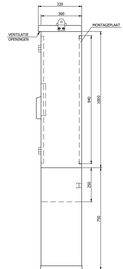
ZIJAANZICHT RECHTS
