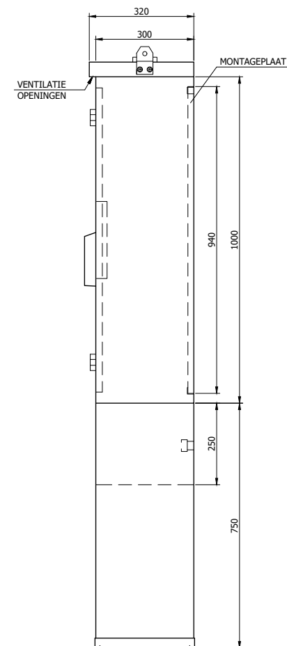
ZIJAANZICHT RECHTS
