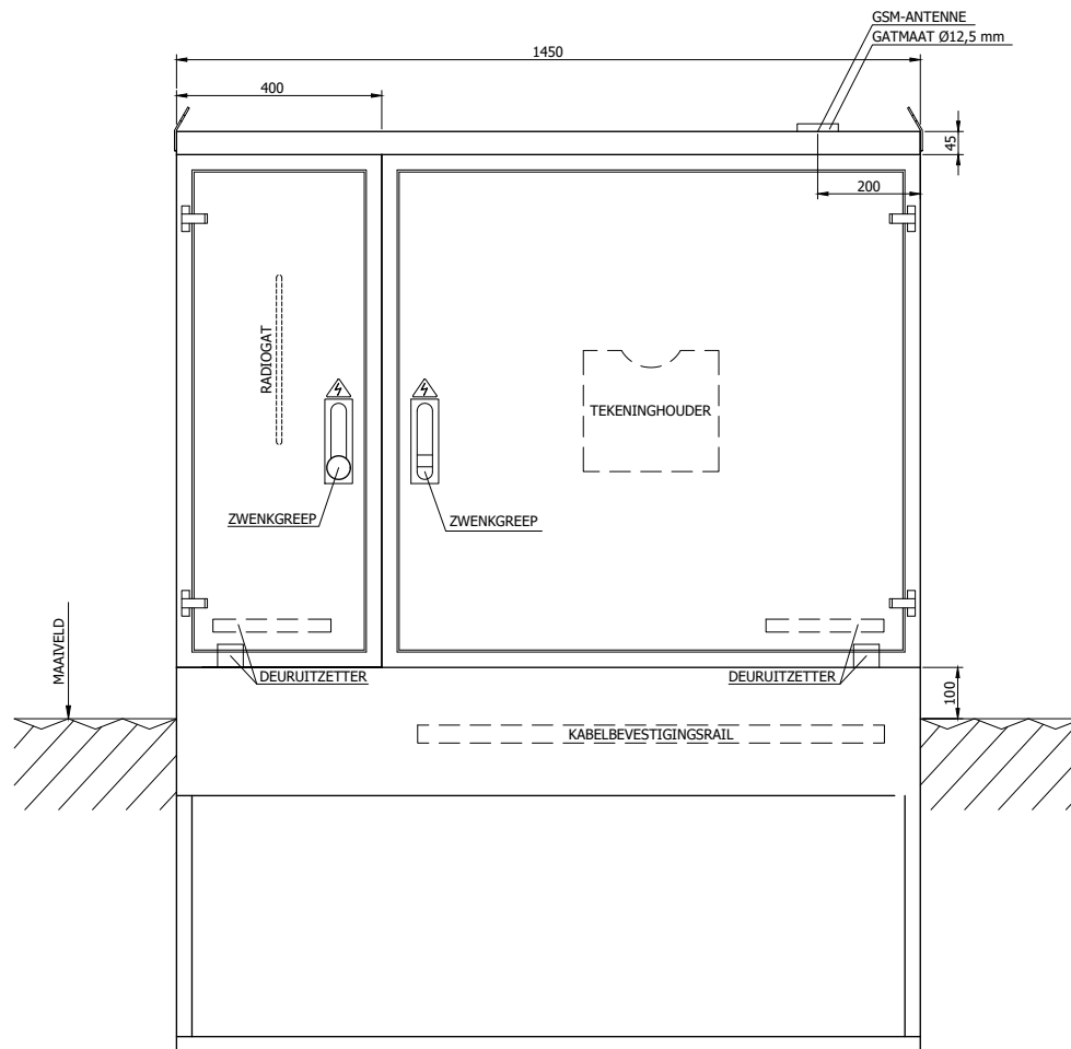
VOORAANZICHT
