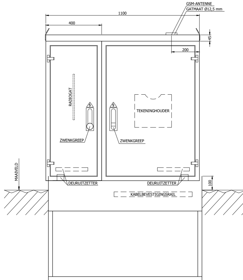
VOORAANZICHT
