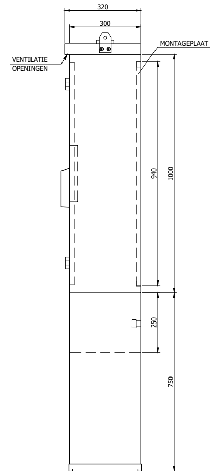
ZIJAANZICHT RECHTS
