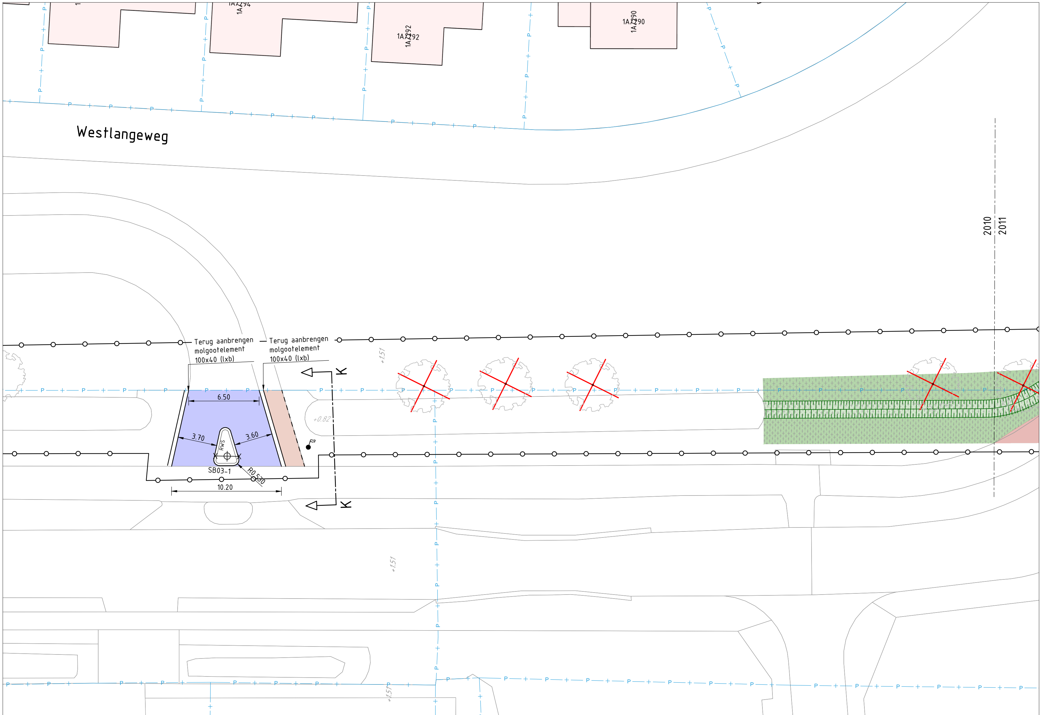
Westlangeweg schaal 1:200
