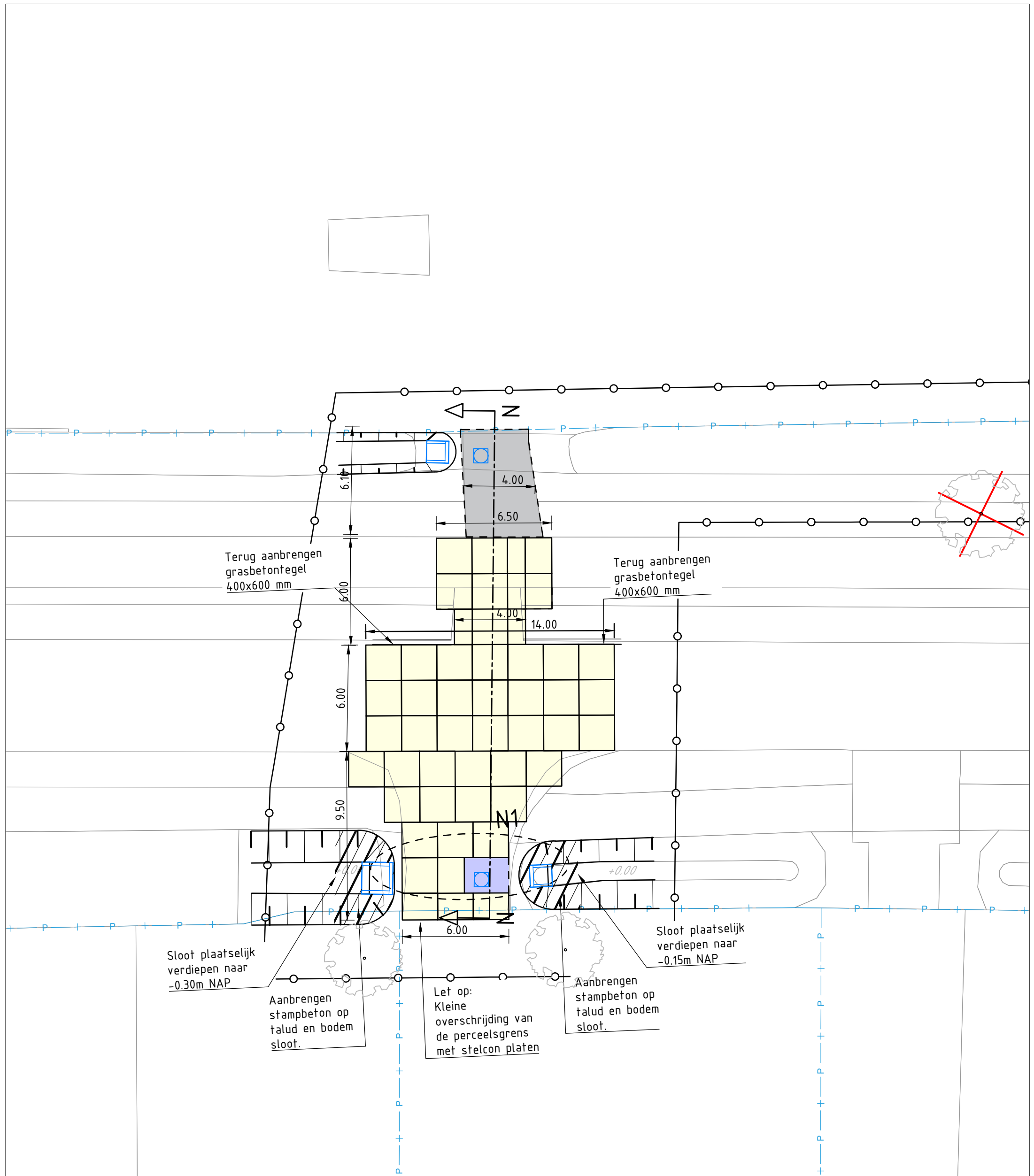
Westlangeweg schaal 1:200
