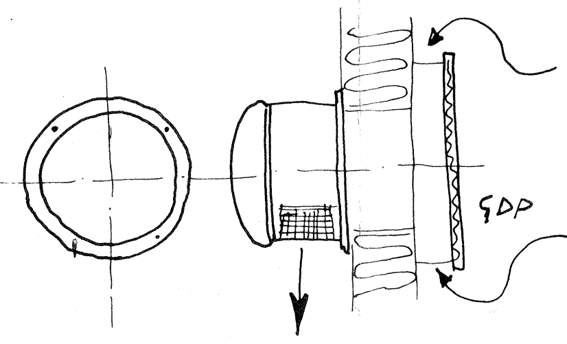
DETAIL DOORSNEDE WAND AFZUIGVENTILATOR
