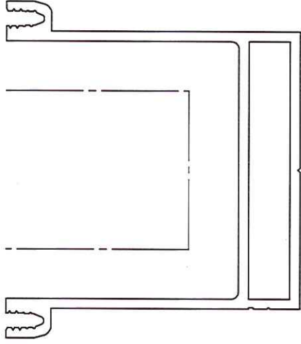
EcoSign Basisprofil Dubbelzijdig gewicht 1369 g/m omtrek 298mm
