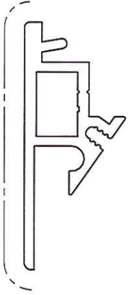
EcoSign Frameprofil Top gewicht 669 g/m omtrek 175mm
