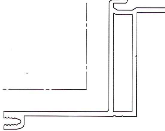
EcoSign Basisprofil Enkelzijdig gewicht 1040 g/m omtrek 298mm
