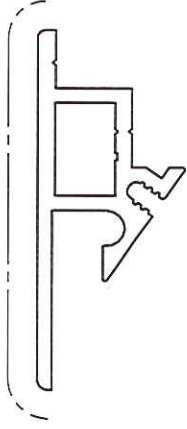
EcoSign Frameprofil gewicht 617 g/m omtrek 175mm
