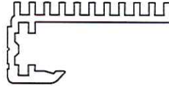
LED profil gewicht 338g/m omtrek 180mm
