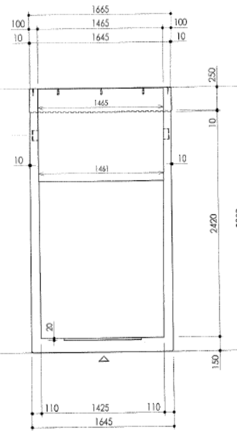
doorsnede B
