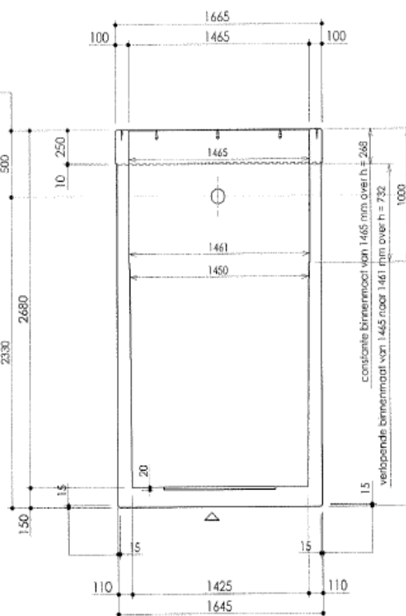
doorsnede A
