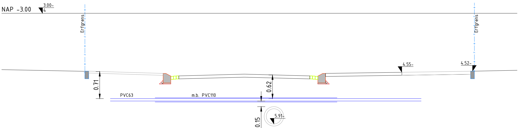
05+06 Kruislaan-Fortweg Schaal 150
