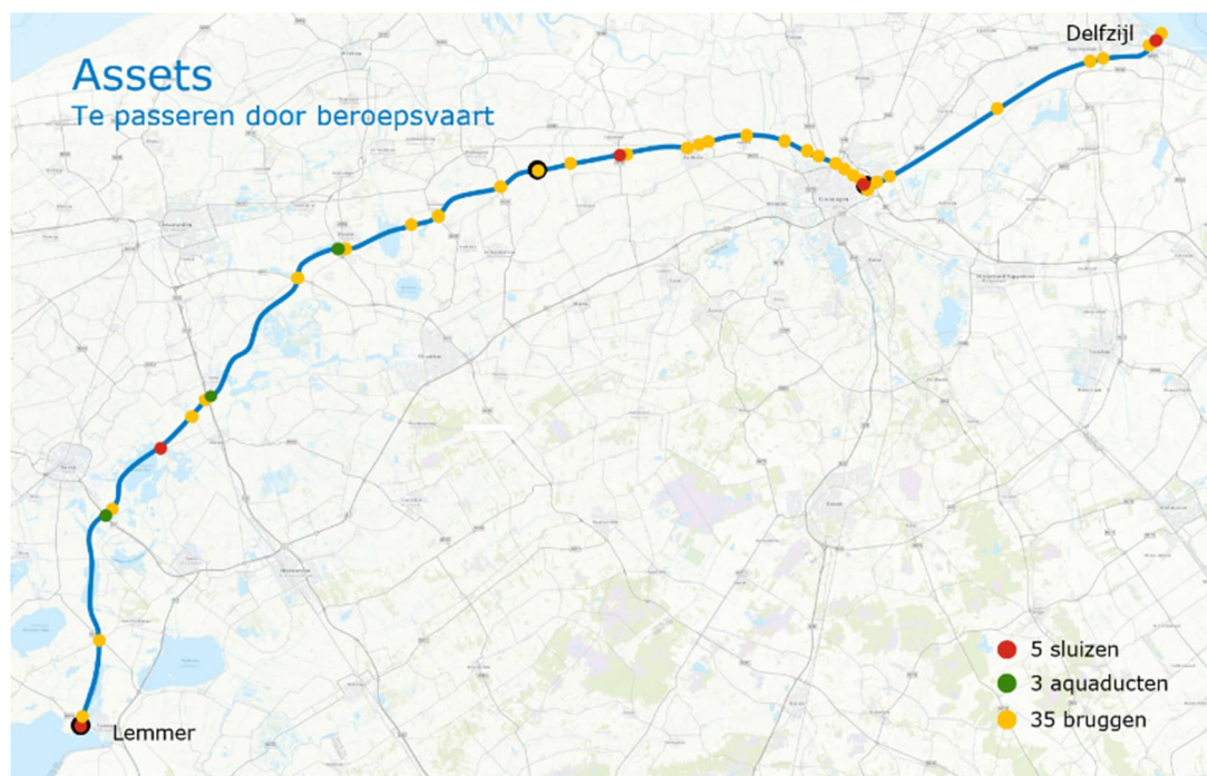
Figuur 2: Grote kunstwerken in de HLD
