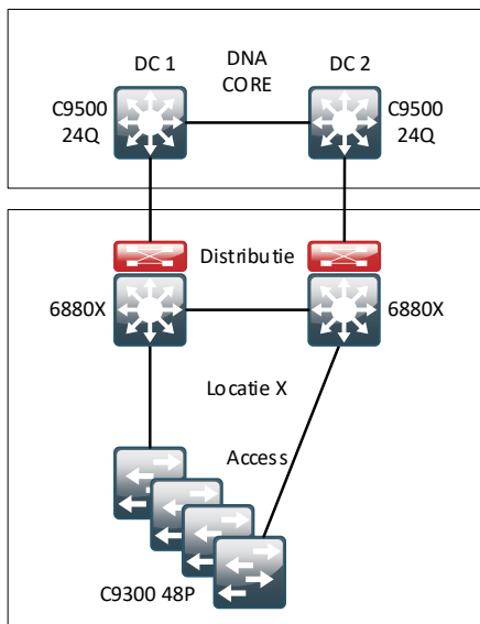
Figuur 2: Configuratie Distributiemodel A
