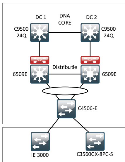
Figuur 8: Configuratie OOV-CAM switches
