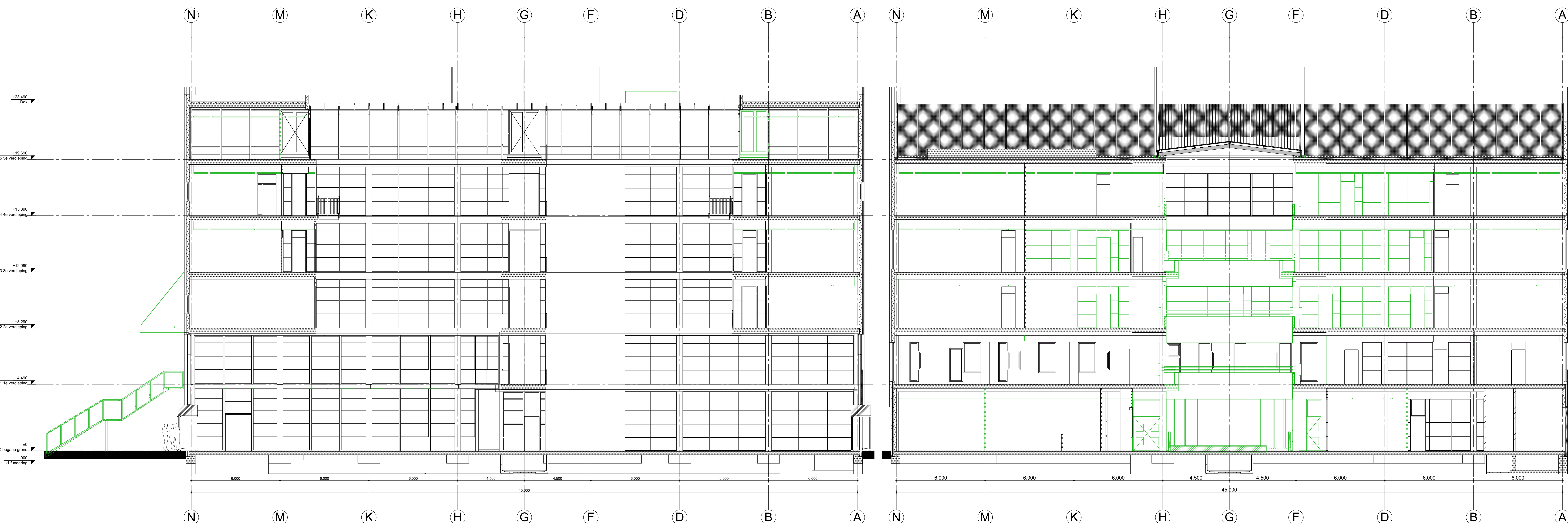
02 doorsnede B-B
