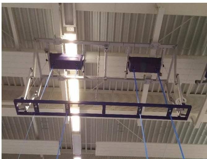
Rekstokinstallatie
