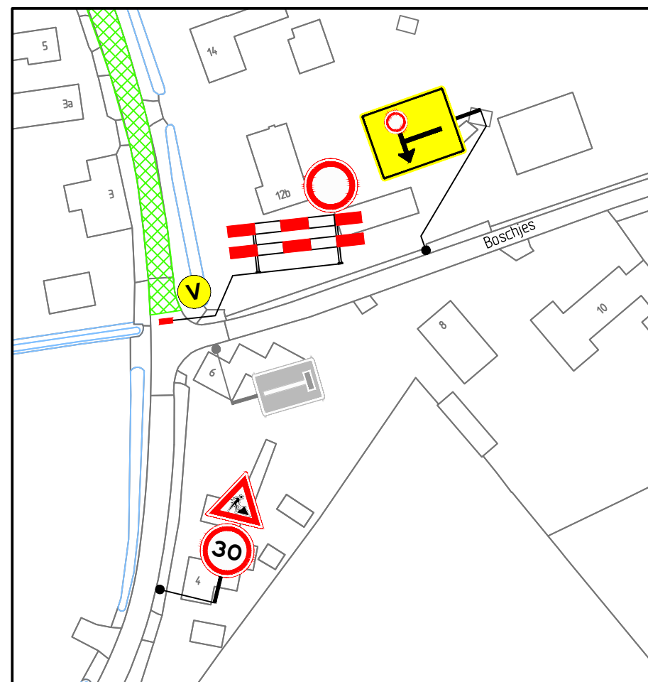
DETAIL 2 SCHAAL 1 : 1000 -
