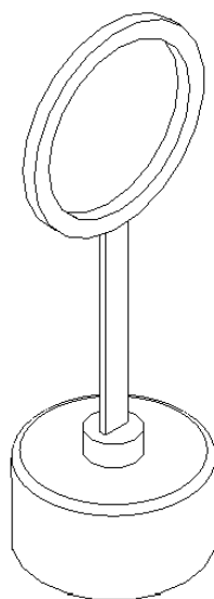
Techno IP66 stekersysteem Afsluitdop IP66 voor T-splitter en eindkabel
