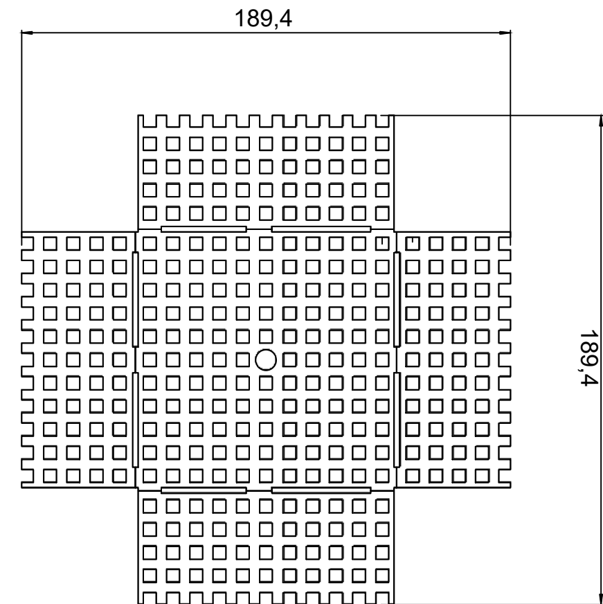
Uitslag schaal 1:2
