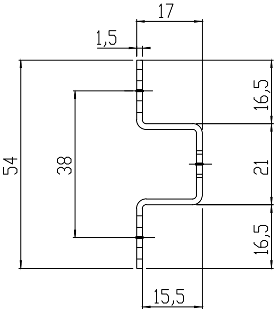
ZET TOLERANTIE: ±0.5
