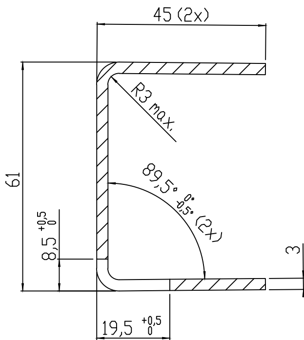
SECTION A-A SCALE 1 : 1
