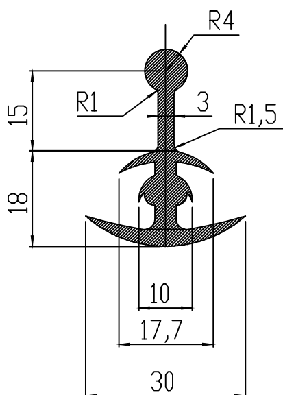
SECTION A-A 1:1
