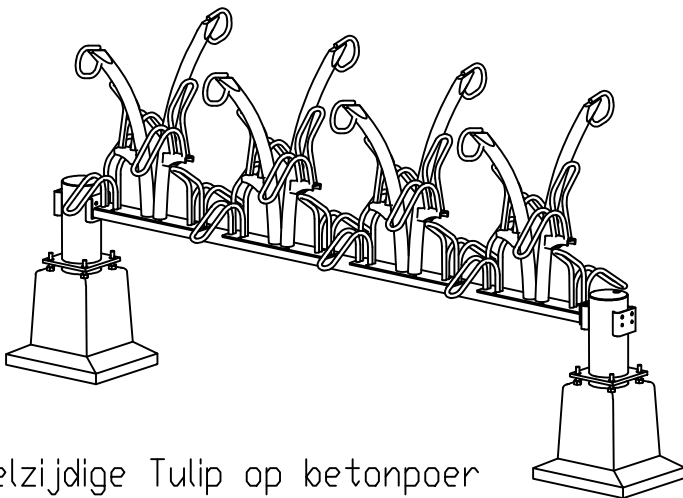
Enkelzijdige Tulip op betonpoer Zie ook tekening 7141-105
