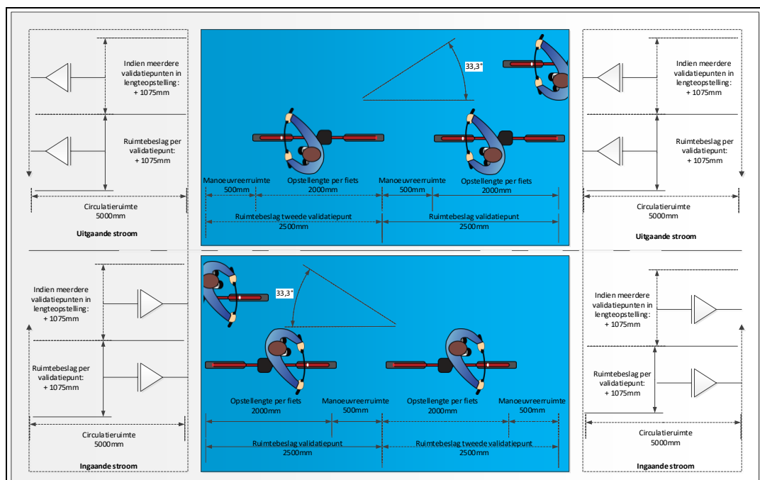
Illustratie: Afmetingen ruimtebeslag validatiesysteem
