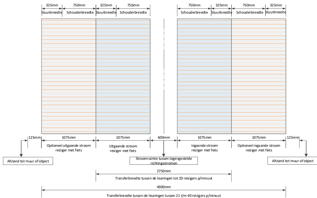
Illustratie: Transferpaden fietsenstalling voor horizontale verplaatsing
