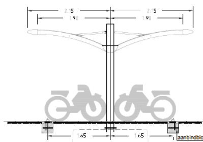
Traverse met kap met nletje - zij aanzicht
