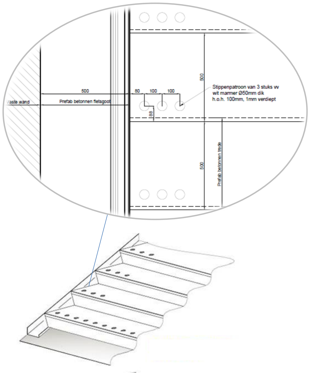
Illustratie: Markering op traptredes
