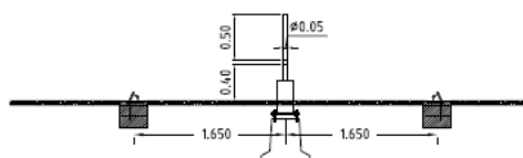
Traverse met nletje - zij aanzicht Schaal 1:50
