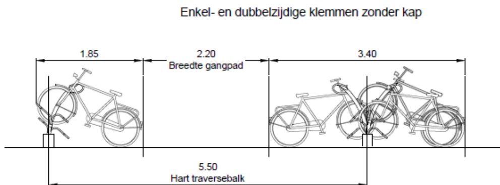
Illustratie: Uitpandige traveemaat bij enkellaags fietsparkeersysteem
