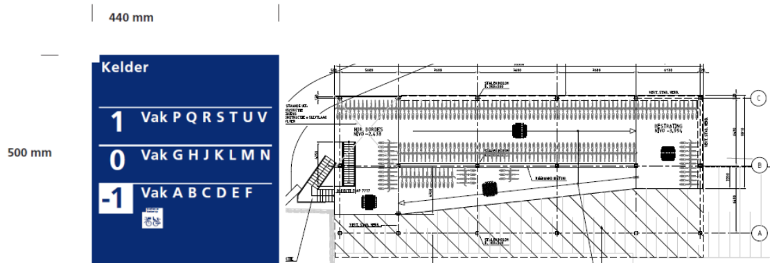
Illustratie: Bewegwijzering vakken HBF-systeem en voorbeeld van de genoemde rekopstelling
