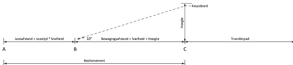
Illustratie: Formule vrijwaarde van beslismoment
