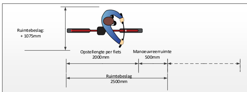
Illustratie: Ruimtebeslag reiziger met fiets
