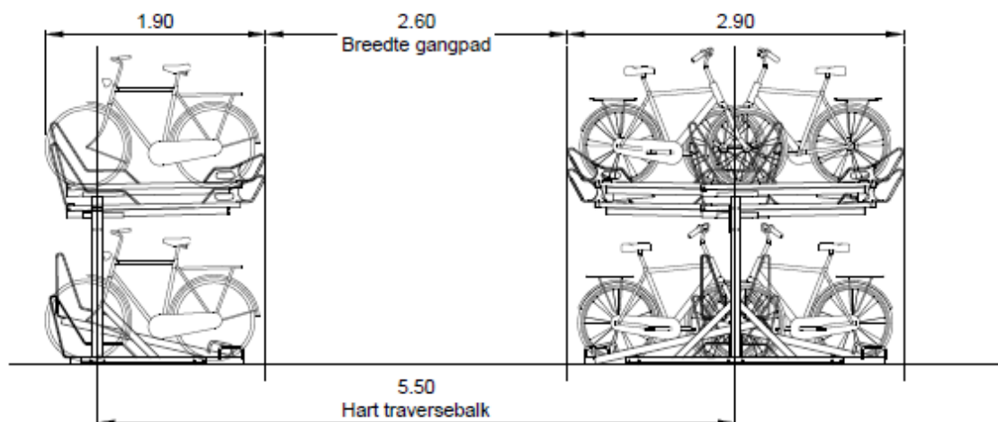
Illustratie: Uitpandige traveemaat bij dubbellaags fietsparkeersysteem
