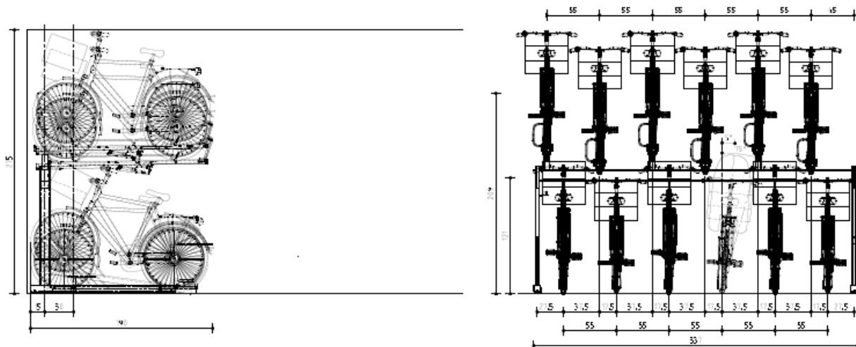
Illustratie: Ruimtebeslag fietsparkeersysteem buitenmodell fietsen
