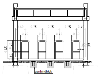
Traverse met kap met nletje - vooraanzicht
