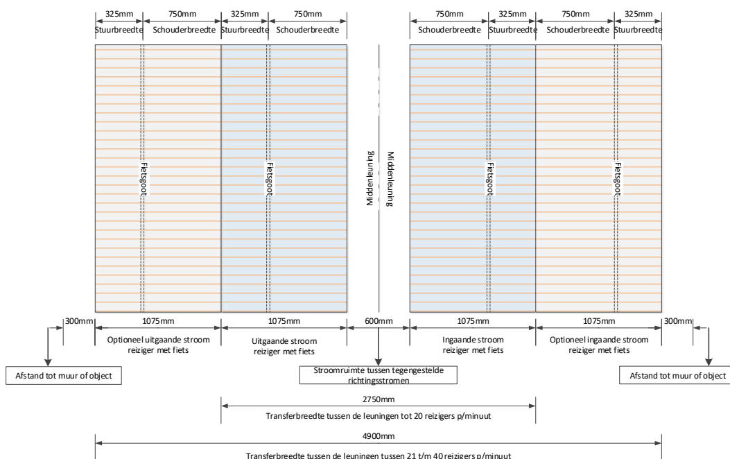
Illustratie: Transferpaden fietsenstalling voor verticale verplaatsing
