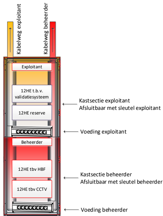
Illustratie: Voorbeeld datakast
