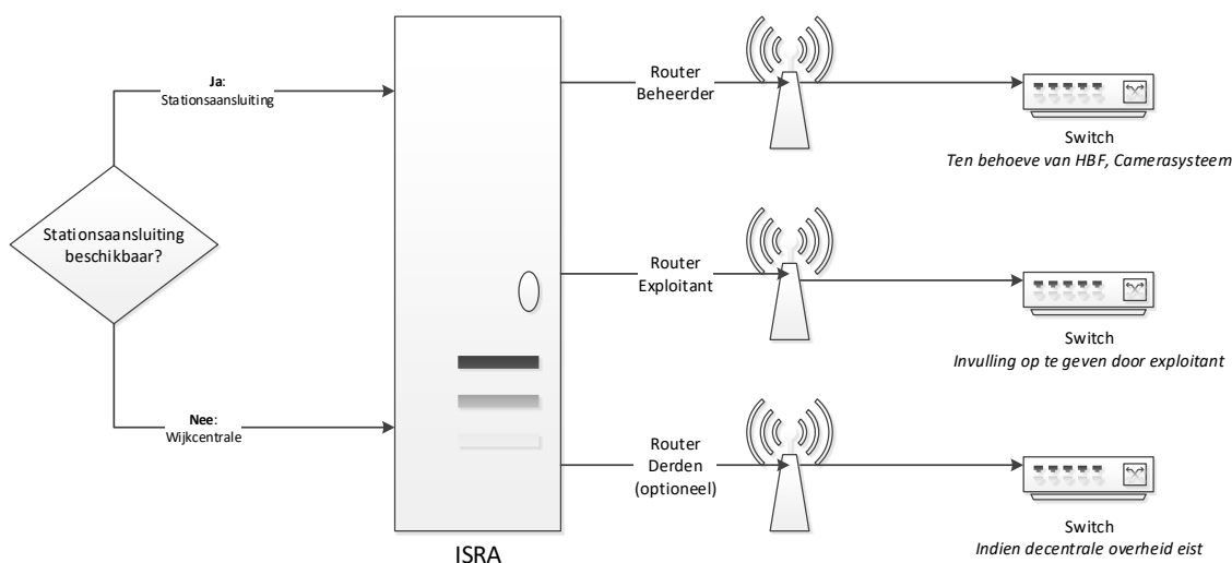
Illustratie: Voorbeeld ISRA-punt
