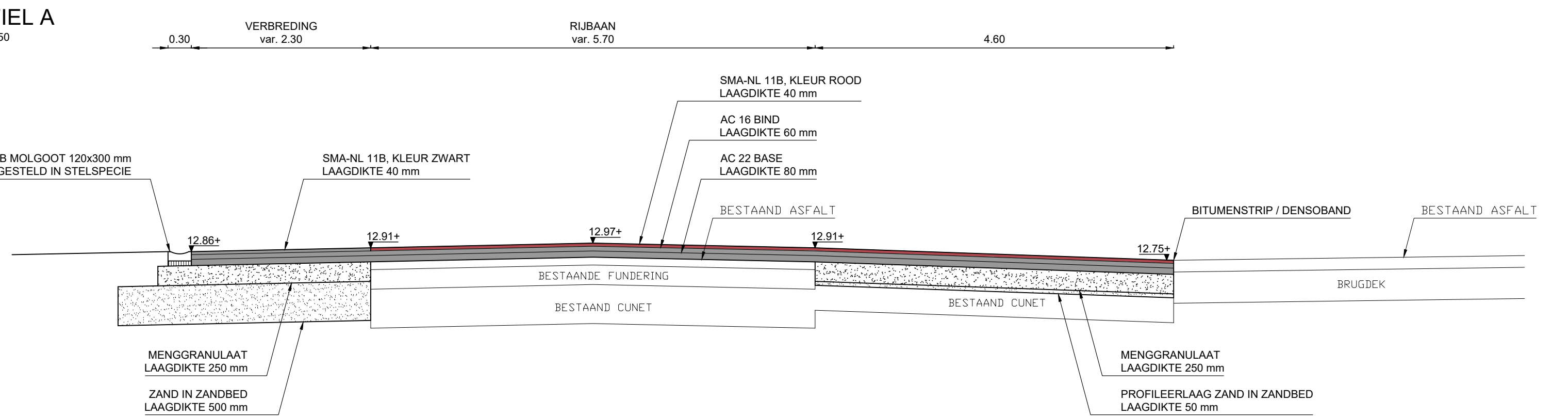
PROFIEL A SCHAAL 1:50
