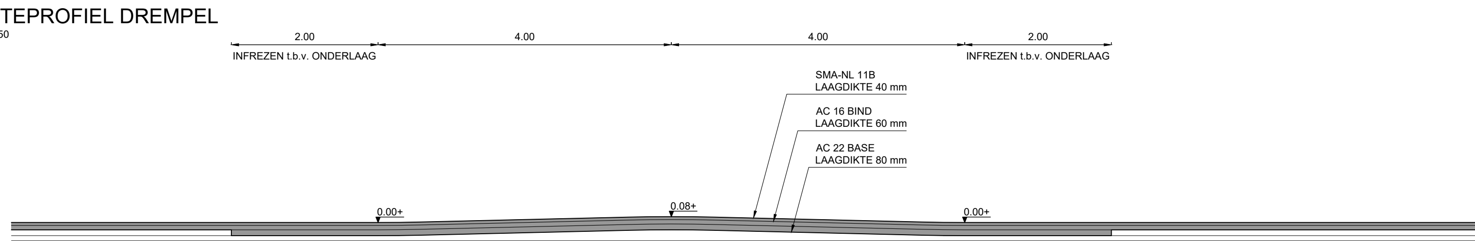
LENGTEPROFIEL DREMPEL SCHAAL 1:50
