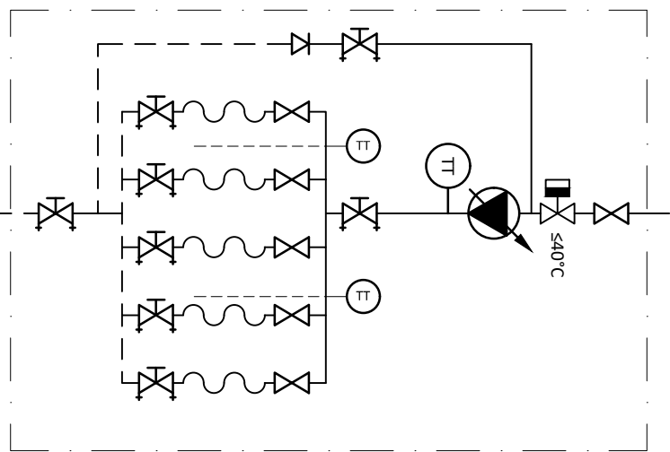
DETAIL VLOERVERWARMING
