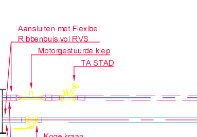
Detail aansluiting koelers
