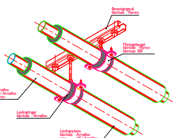
Montage leidingwerk aan plafond
