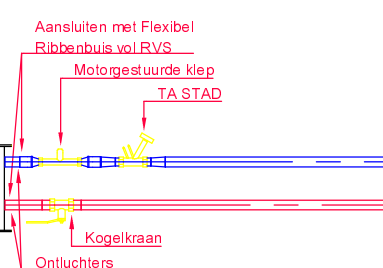
Detail aansluiting verwarmers
