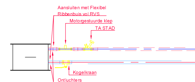
Detail aansluiting koelers
