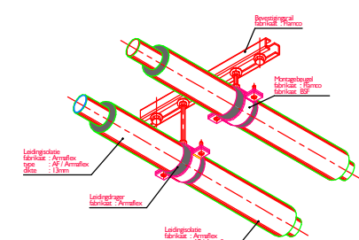
Montage leidingwerk aan plafond
